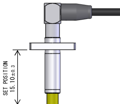
Figure.7 設置寸法 Mounting dimensions
