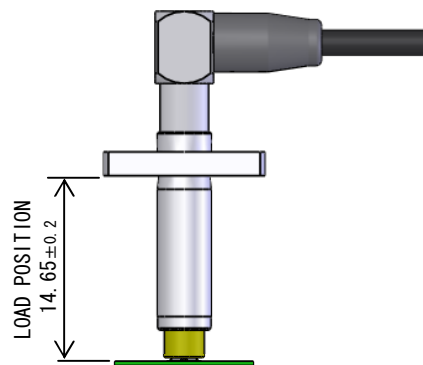
Figure.8 検査寸法 Inspection dimensions
