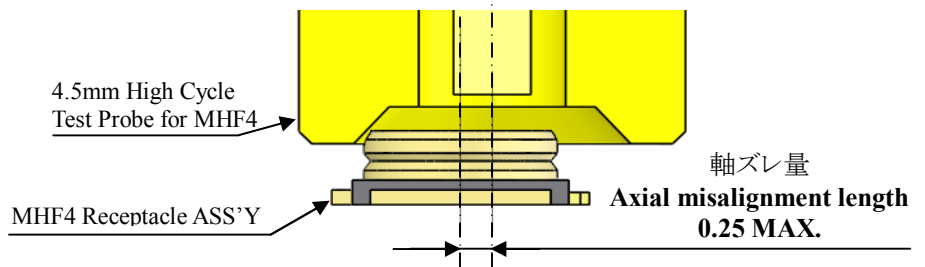
Figure.10 許容誘い込み量 Allowable axial misalignment length
