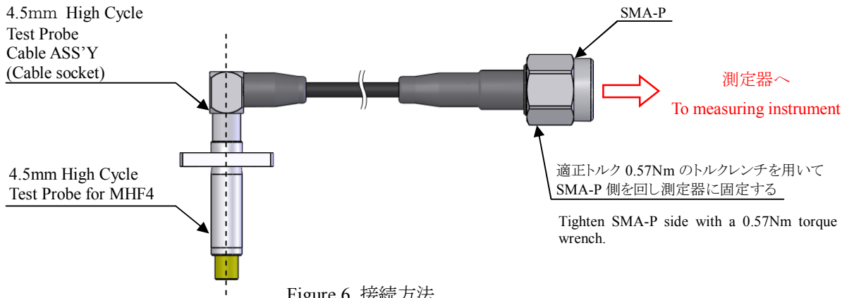
Figure.6 接続方法 Connection method
