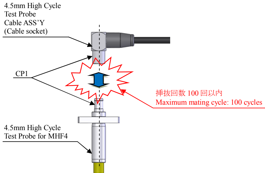
Figure.5 挿抜回数 Mating cycle
