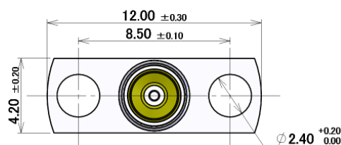
Figure.2 フランジ寸法 Flange dimensions
