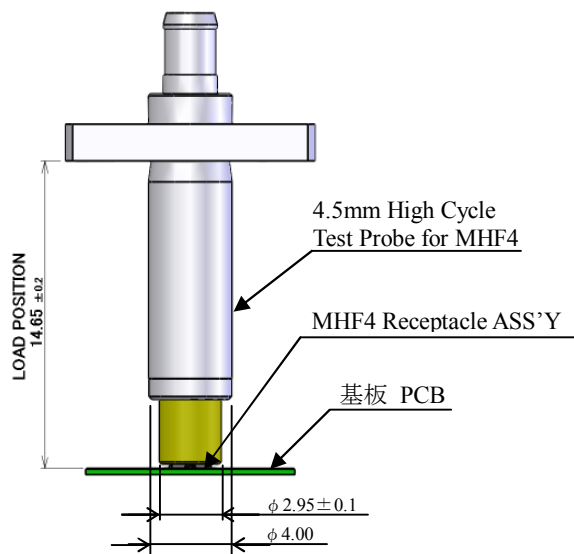
Figure.3 高さ寸法 Height dimension
