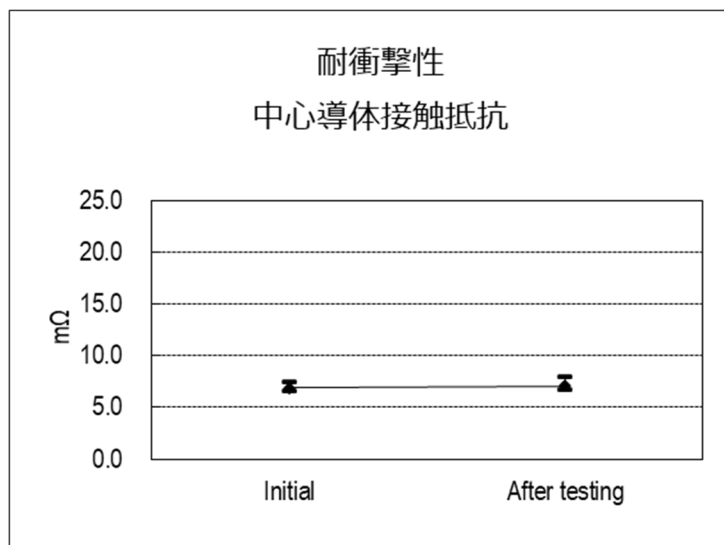
(グラフ 6) 耐衝撃性
