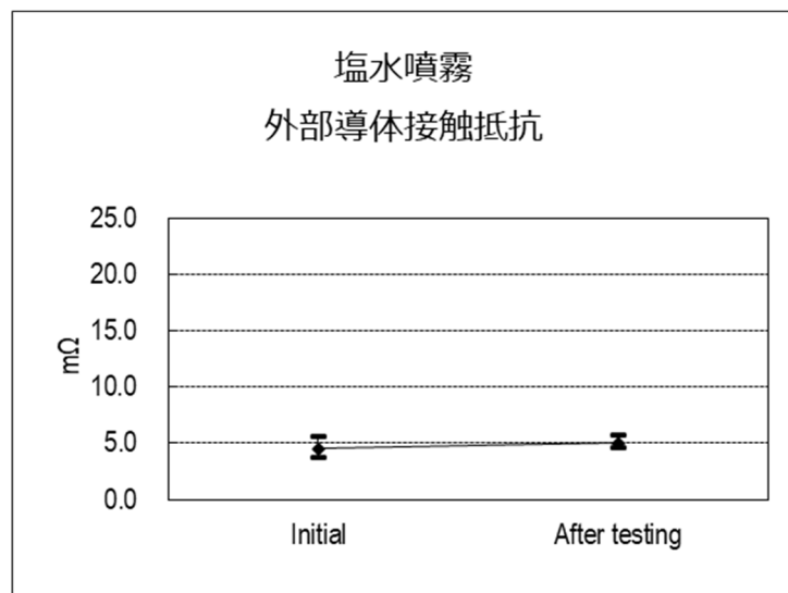
(グラフ 9) 塩水噴霧
