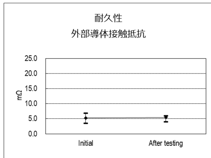
(グラフ 3) 耐久性
