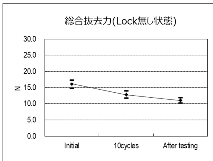
(グラフ 2) 抜去力
