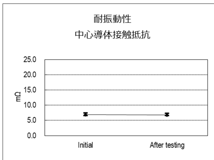
(グラフ 5) 耐振動性
