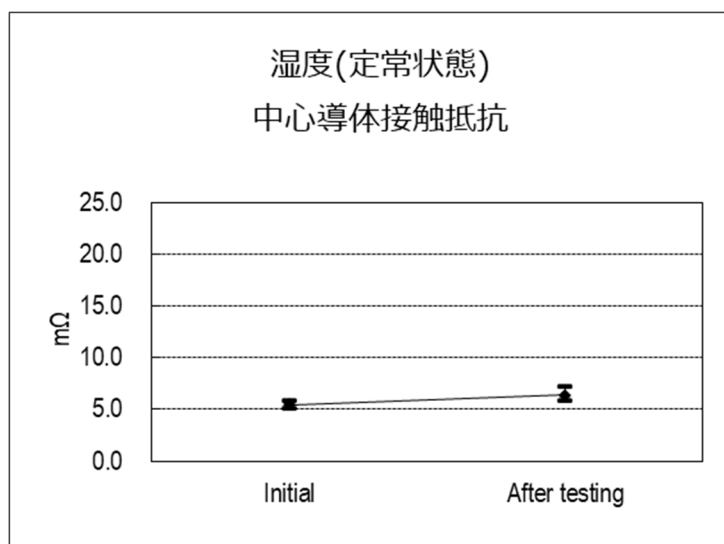
(グラフ 8) 湿度 (定常状態)
