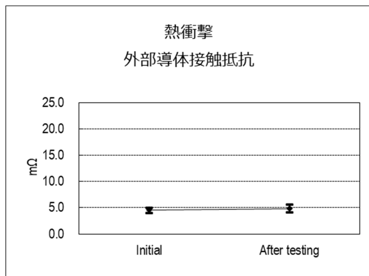
(グラフ 7) 熱衝撃
