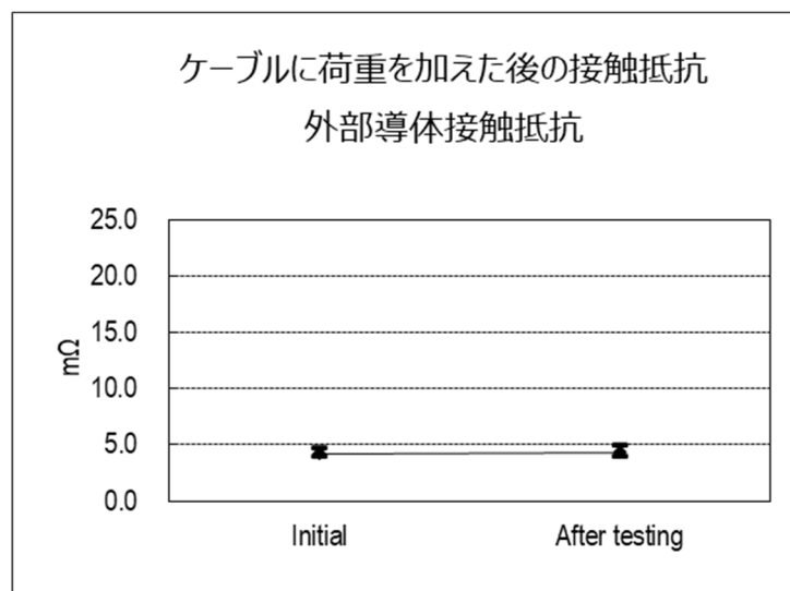
(グラフ 4) ケーブルに荷重を加えた後の接触抵抗
