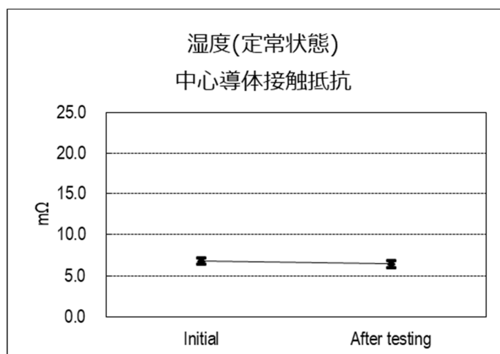
(グラフ 8) 湿度 (定常状態)
