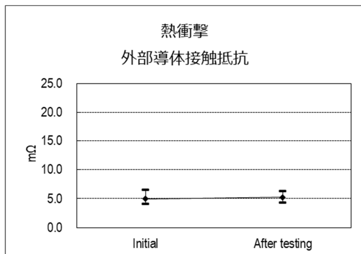
(グラフ 7) 熱衝撃
