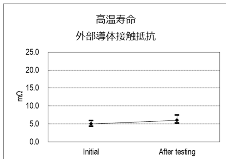
(グラフ 10) 高温寿命
