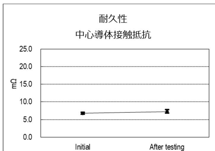
(グラフ 3) 耐久性
