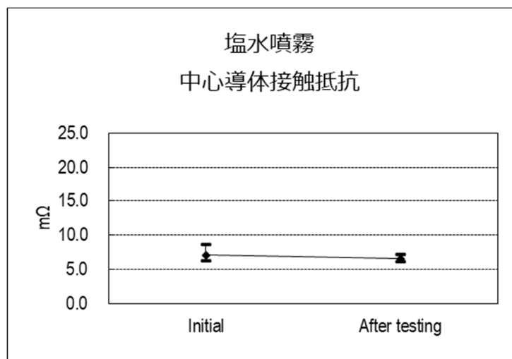
(グラフ 9) 塩水噴霧
