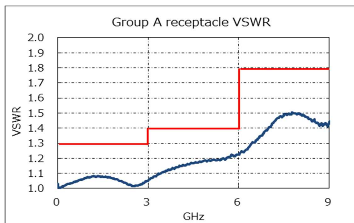
(グラフ 1) 電圧定在波比
