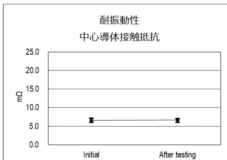
(グラフ 5) 耐振動性
