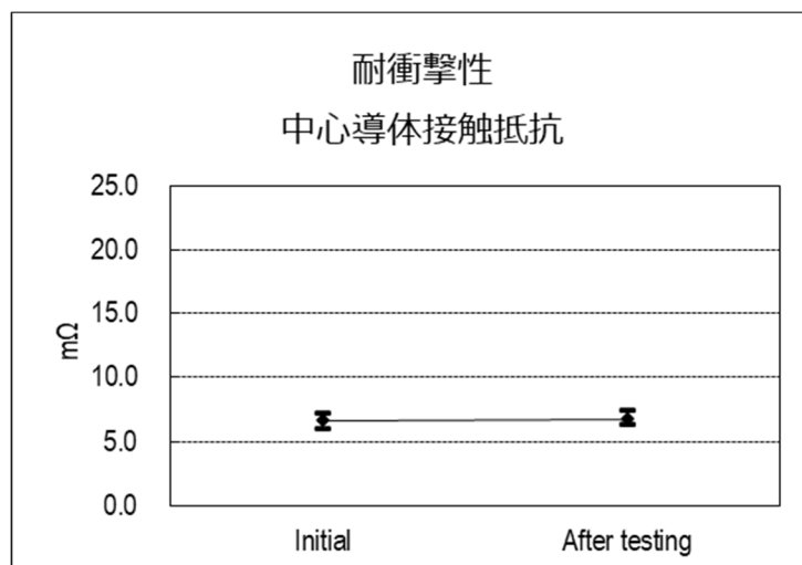
(グラフ 6) 耐衝撃性
