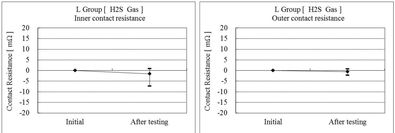
Graph 9 硫化水素ガス
