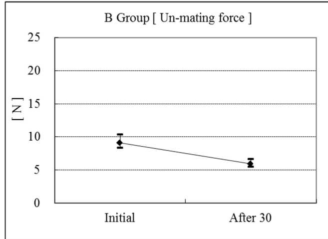
Graph 2 抜去力
