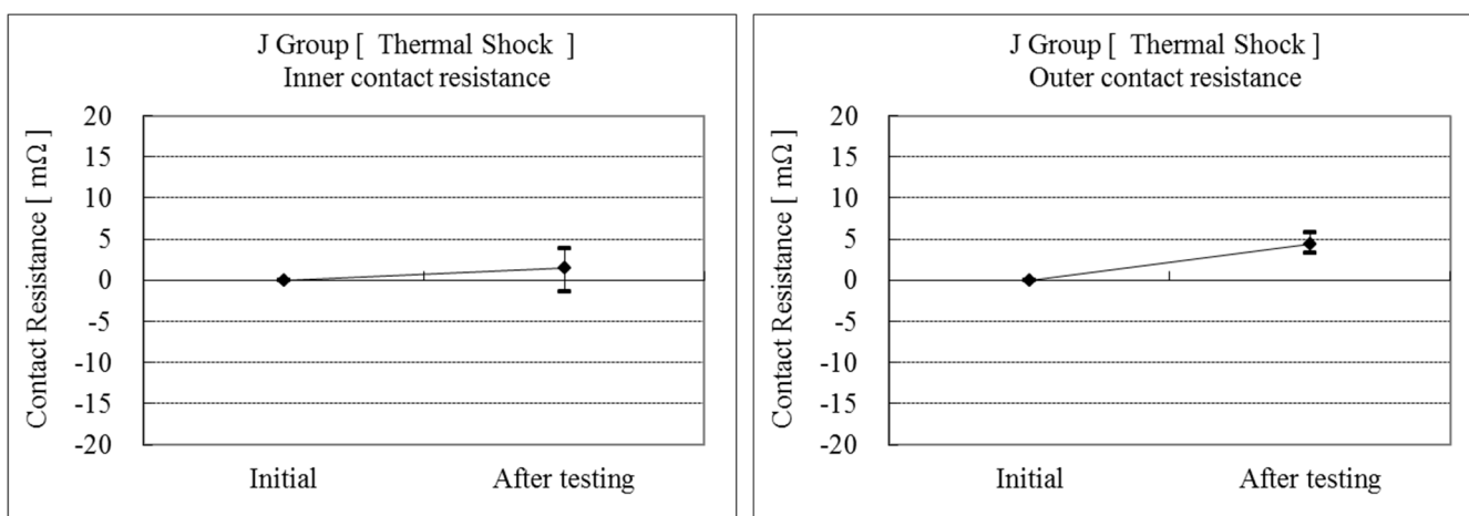
Graph 7 熱衝撃
