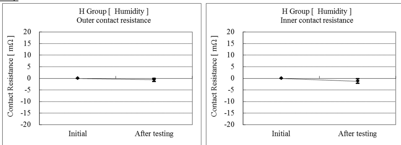
Graph 6 湿度 (定常状態)
