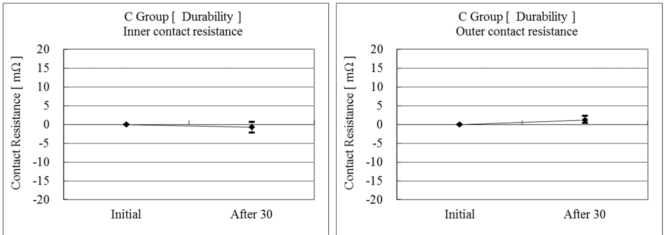
Graph 3 耐久性
