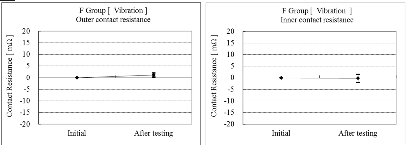
Graph 4 耐振動性
