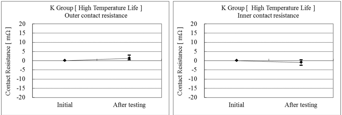
Graph 8 高温寿命
