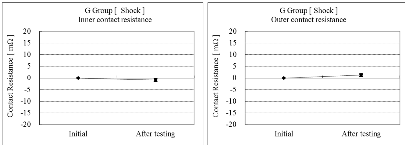
Graph 5 耐衝撃性
