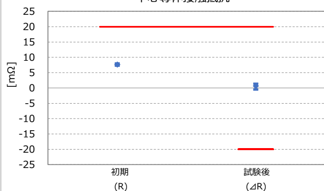
塩水噴霧 Part No. 20565-001R-13 中心導体接触抵抗
