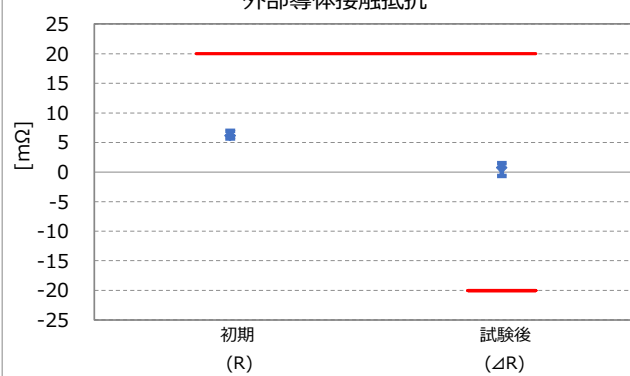
塩水噴霧 Part No. 20572-001R-08 外部導体接触抵抗
