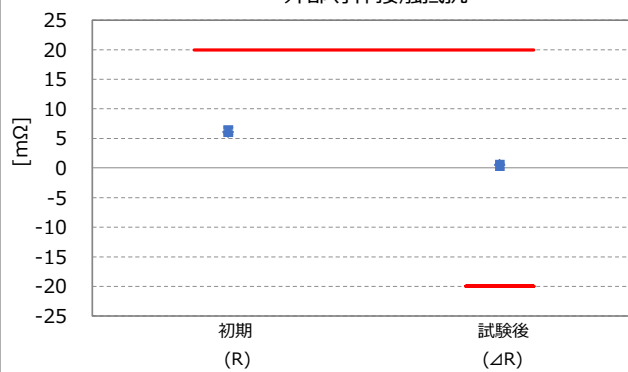
耐衝撃性 Part No. 20565-001R-13 外部導体接触抵抗
