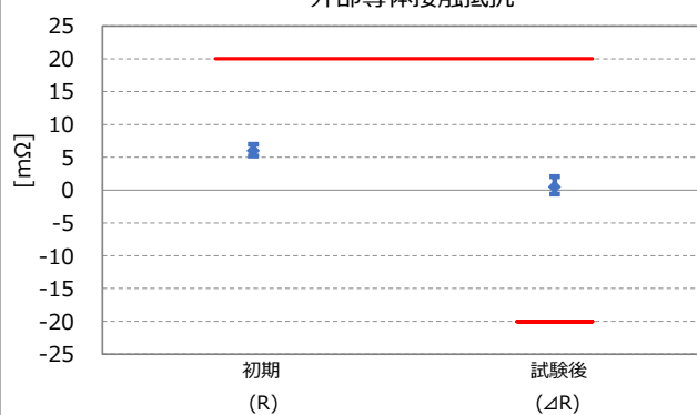
耐衝撃性 Part No. 20572-001R-08 外部導体接触抵抗
