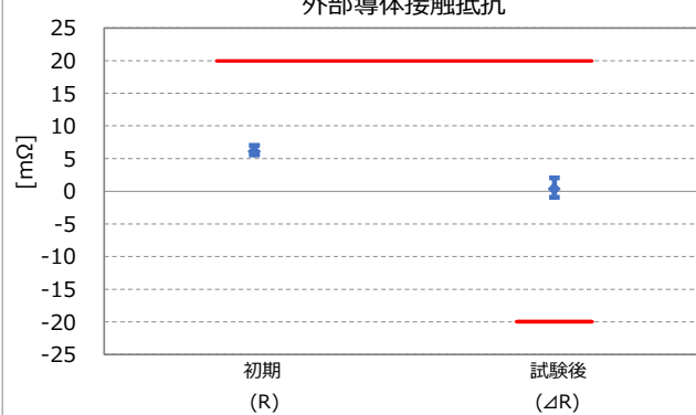
硫化水素ガス Part No. 20565-001R-13 外部導体接触抵抗
