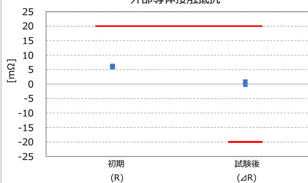
塩水噴霧 Part No. 20565-001R-13 外部導体接触抵抗
