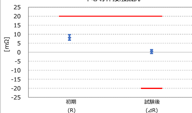
硫化水素ガス Part No. 20565-001R-13 中心導体接触抵抗
