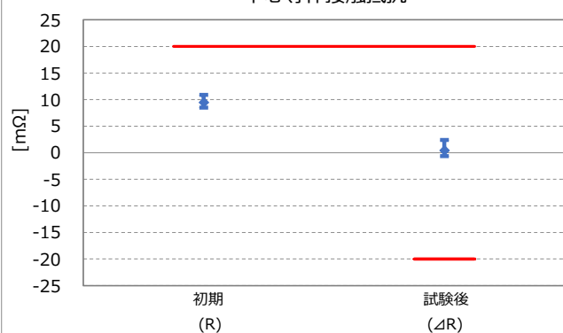
塩水噴霧 Part No. 20572-001R-08 中心導体接触抵抗
