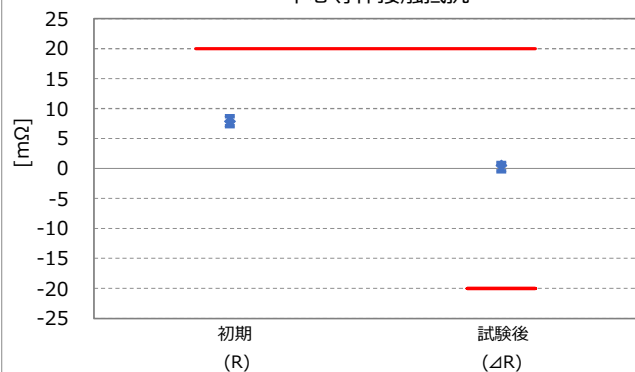
耐衝撃性 Part No. 20565-001R-13 中心導体接触抵抗
