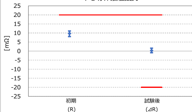
耐振動性 Part No. 20572-001R-08 中心導体接触抵抗
