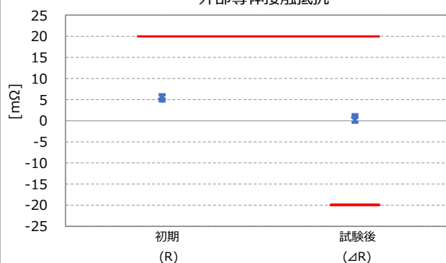
耐振動性 Part No. 20572-001R-08 外部導体接触抵抗
