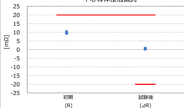
耐衝撃性 Part No. 20572-001R-08 中心導体接触抵抗
