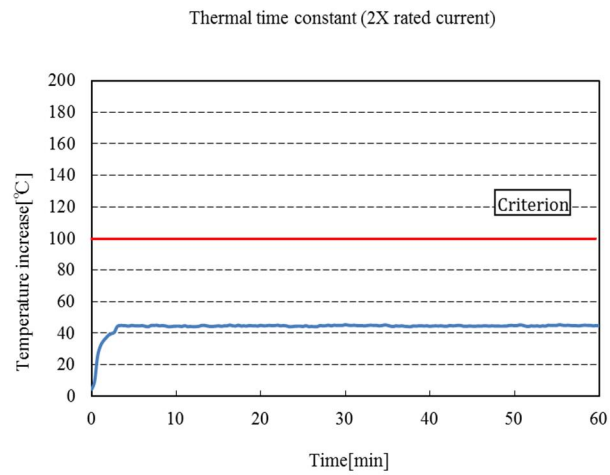
Graph 20. PG14 E14.1 Thermal time constant
