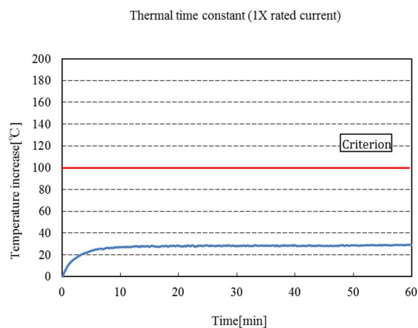
Graph 24. PG14 E14.1 Thermal time constant
