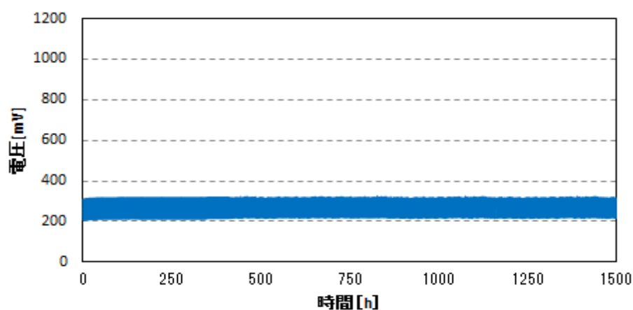
グラフ 2. サーマルショック 抵抗変動モニタ
