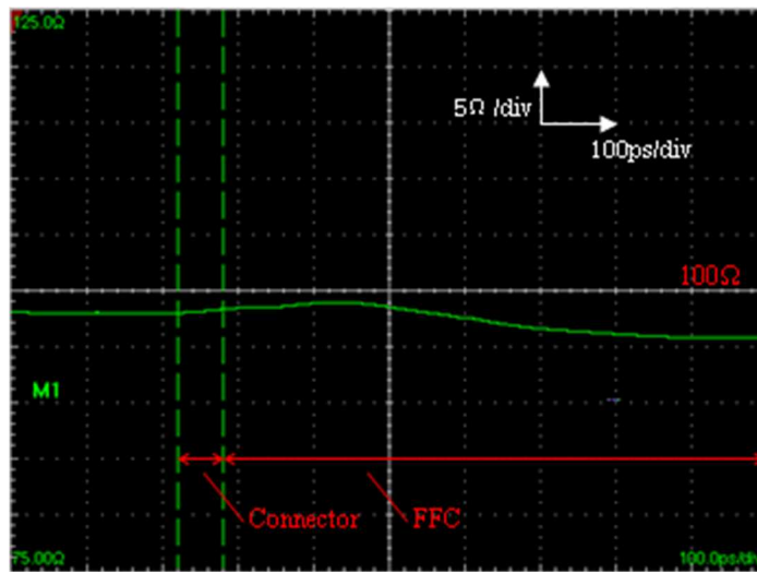
Graph.1 差動インピーダンス/Differential Impedance
