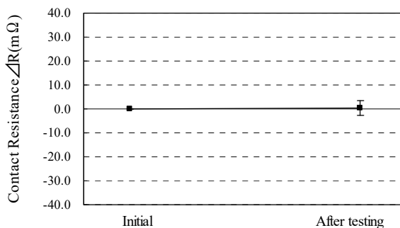
Graph.7 接触抵抗の変化：高温寿命
