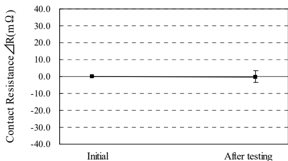
Graph.8 接触抵抗の変化：湿度（定常状態）
