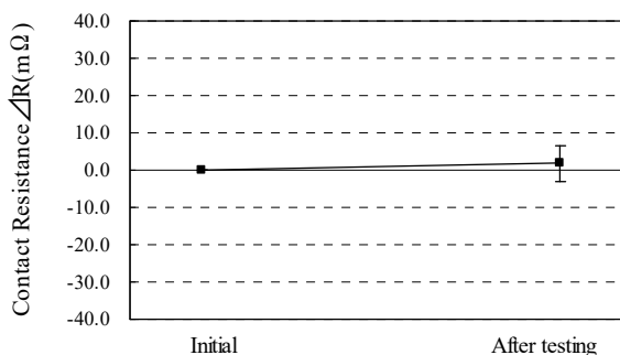
Graph.11 接触抵抗の変化：ガス (H 2 S)
