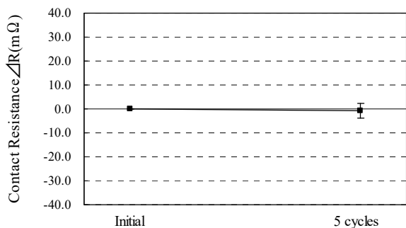
Graph.6 接触抵抗の変化：熱衝撃
