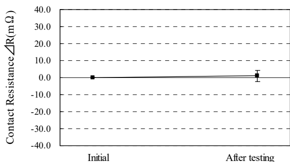
Graph.10 接触抵抗の変化：塩水噴霧
