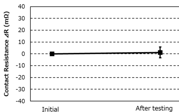
グラフ 8. 接触抵抗の変化 (Kグループ : 湿度(定常状態))
