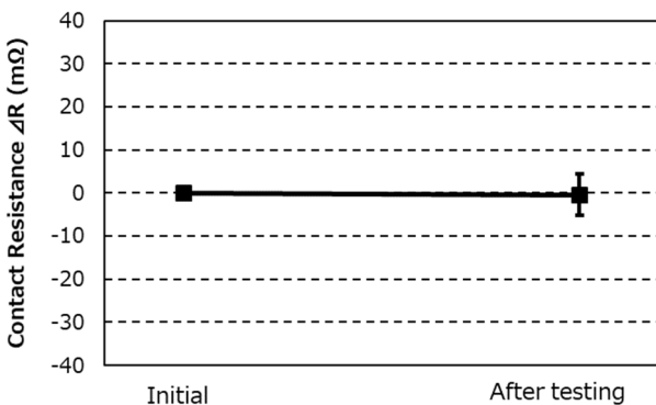
グラフ 5. 接触抵抗の変化 (Gグループ：熱衝撃)
