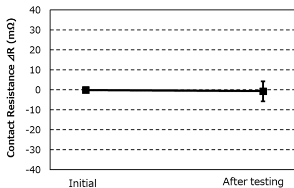
グラフ 8. 接触抵抗の変化 (Kグループ : 湿度(サイクリング))
