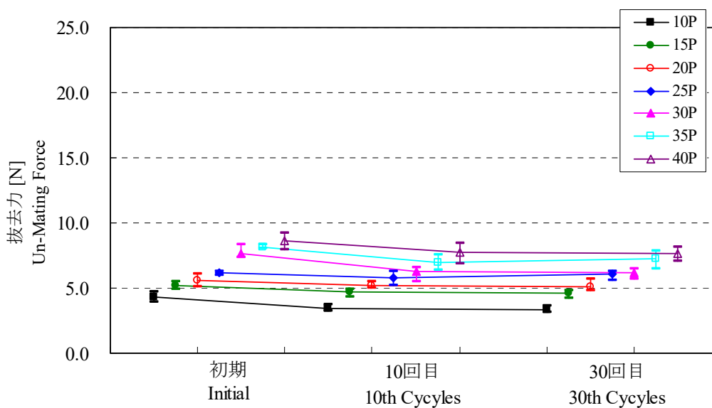
Graph 2. ロック無 抜去力の変化
