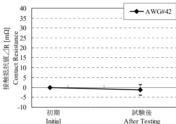
Graph 9. AWG#42 接触抵抗値の変化 Dグループ: 熱衝撃 A change of contact resistance D group : Thermal Shock
