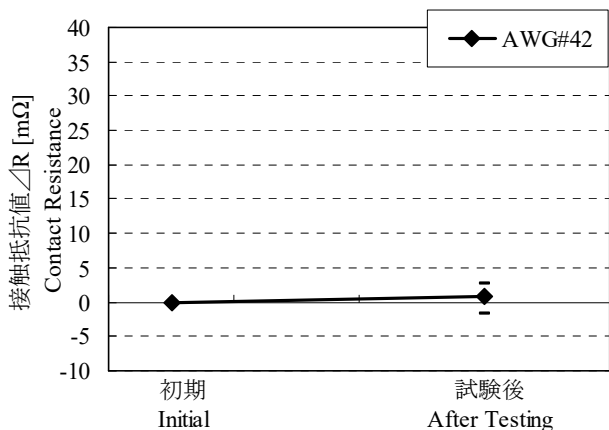
Graph 5. AWG#42 接触抵抗値の変化 A グループ: 耐久性 A change of contact resistance A group : Durability
