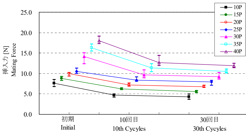
Graph 1. ロック無 挿入力の変化
