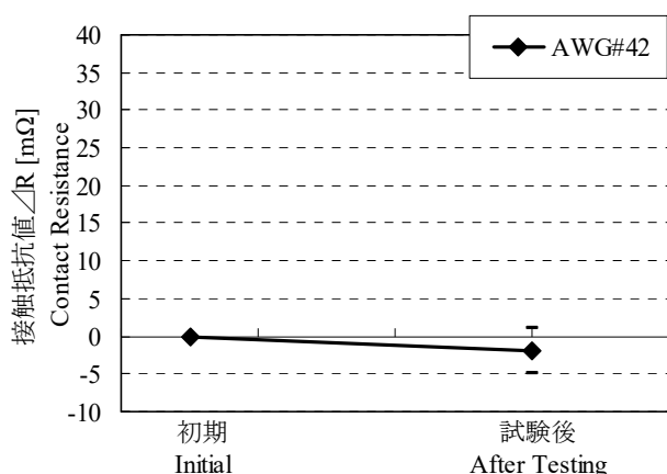
Graph 15. AWG#42 接触抵抗値の変化 Gグループ:湿度(サイクリング) A change of contact resistance G group : Humidity (Cycling)
