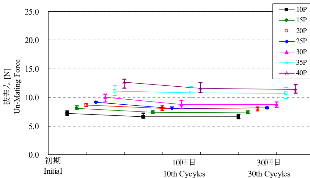
Graph 4. ロック有 抜去力の変化 Aグループ:抜去力 A chnge of UNmatingForce With Lock/ A Group : UnmatingForce
