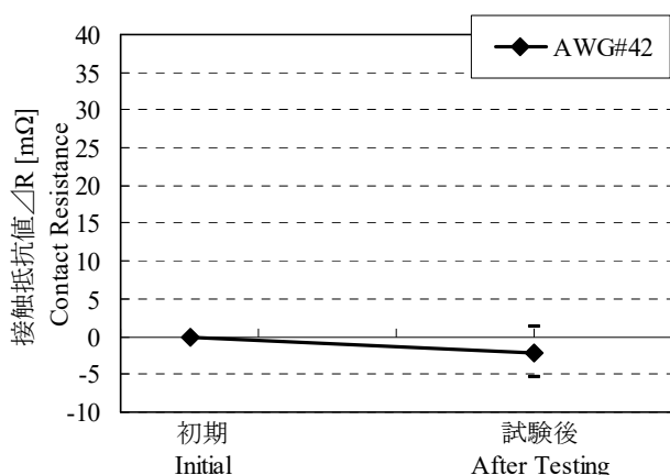
Graph 13. AWG#42 接触抵抗値の変化 Fグループ:湿度(定常状態) A change of contact resistance F group : Humidity (Steady State)
