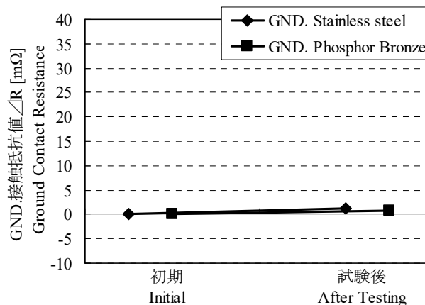
Graph 6. GND 接触抵抗値の変化 A グループ: 耐久性 A change of ground contact resistance A group : Durability
