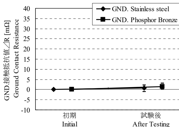
Graph 10. GND 接触抵抗値の変化 Dグループ: 熱衝撃 A change of ground contact resistance D group : Thermal Shock
