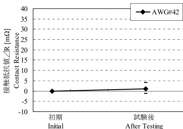
Graph 11. AWG#42 接触抵抗値の変化 Eグループ: 高温寿命 A change of contact resistance E group : High Temp. Life
