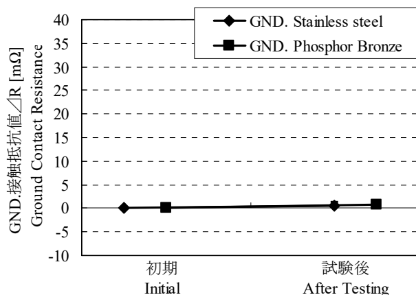
Graph 12. GND 接触抵抗値の変化 Eグループ: 高温寿命 A change of ground contact resistance E group : High Temp. Life
