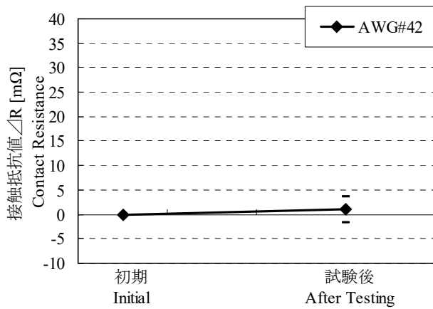
Graph 17. AWG#42 接触抵抗値の変化 Hグループ: 塩水噴霧 A change of contact resistance H group : Salt Water Spray
