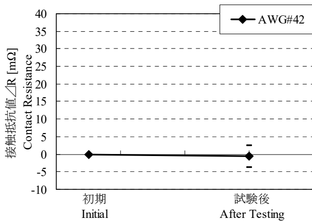
Graph 19. AWG#42 接触抵抗値の変化 Jグループ: ガス(H 2 S) A change of contact resistance J group : Gas (H 2 S)
