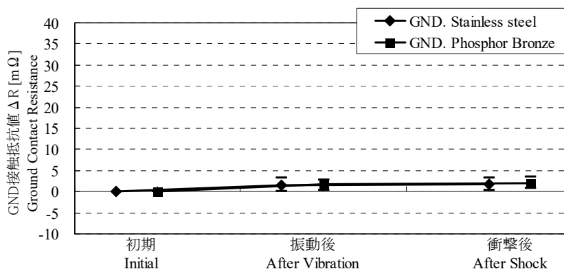
Graph 8. GND 接触抵抗値の変化 C グループ: 振動・衝撃 A change of ground contact resistance C group : Vibration / Shock
