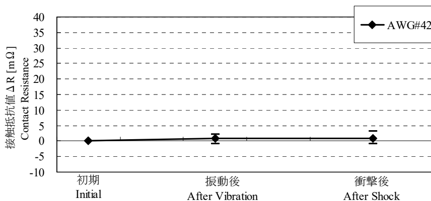
Graph 7. AWG#42 接触抵抗値の変化 C グループ: 振動・衝撃 A change of contact resistance C group : Vibration / Shock
