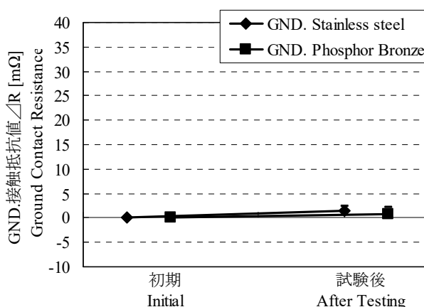
Graph 16. GND 接触抵抗値の変化 Gグループ:湿度サイクル A change of ground contact resistance G group : Humidity Cycle
