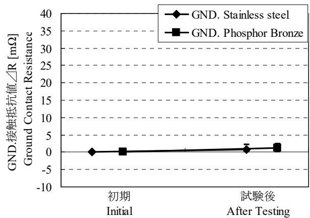
Graph 20. GND 接触抵抗値の変化 Jグループ: ガス(H 2 S) A change of ground contact resistance J group : Gas (H 2 S)
