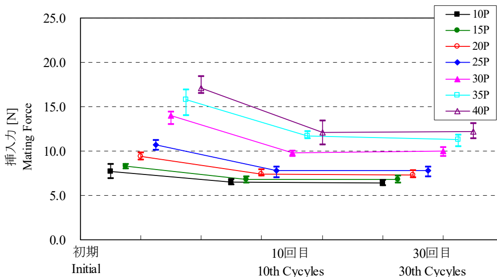
Graph 3. ロック有 挿入力の変化 Aグループ:挿入力 A chnge of MatingForce With Lock / A Group : MatingForce
