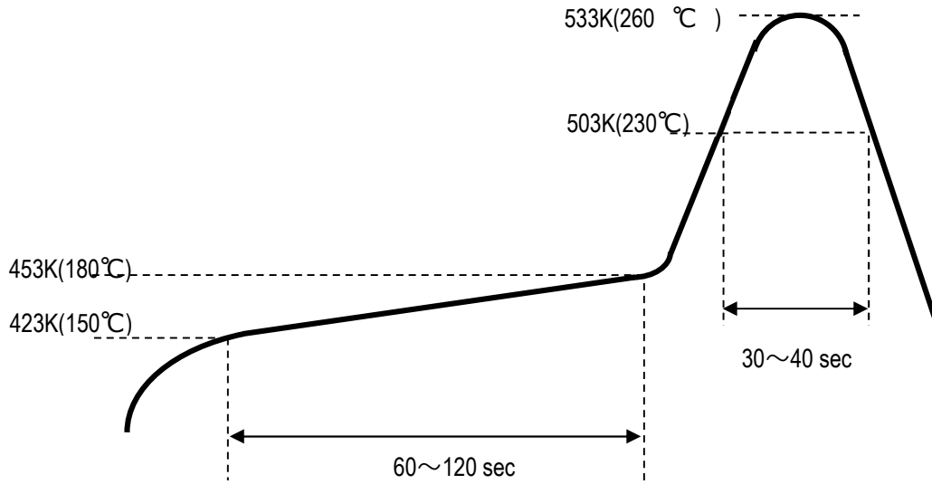
図. 1 リフロープロフィール
