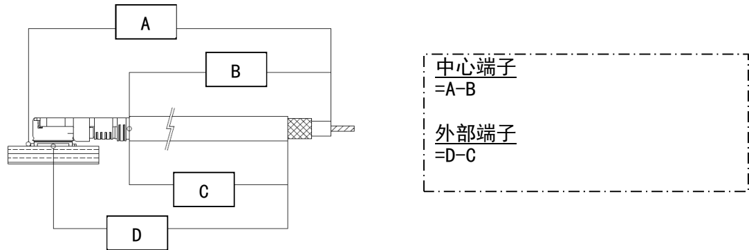
图 1 接触电阻
