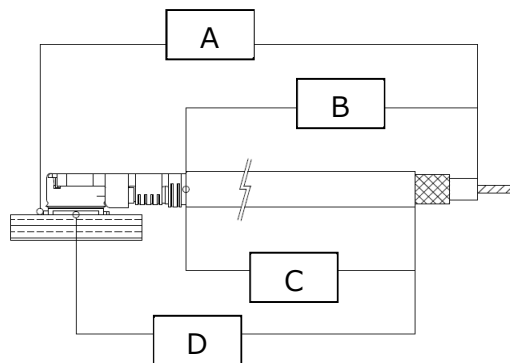
图 1 接触电阻
