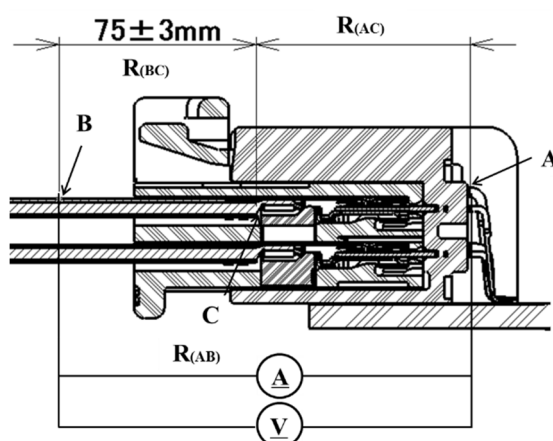
図 2.接続回路及び測定位置
