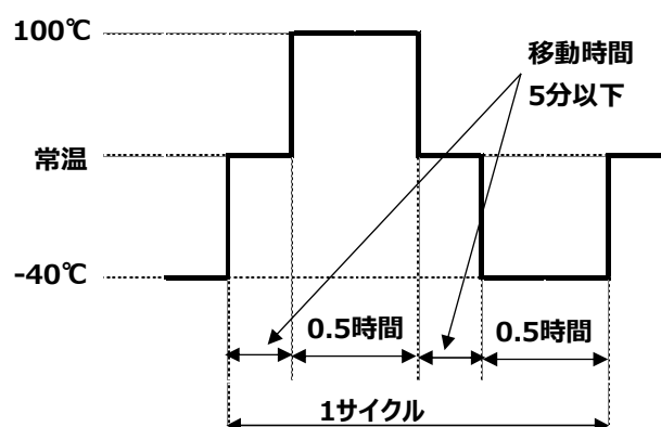
図 3.サーマルショック
