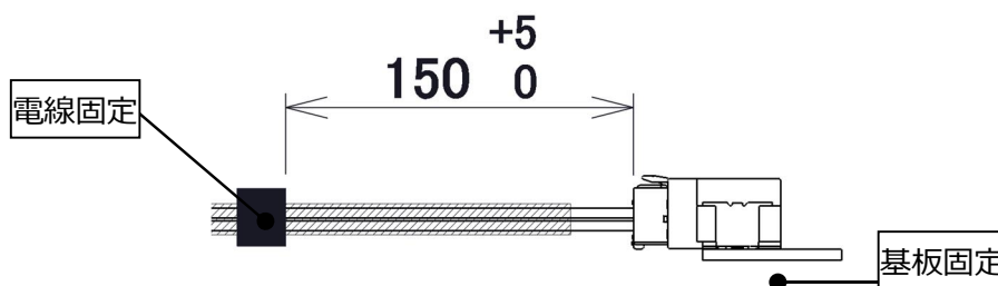
図 8.固定方法
