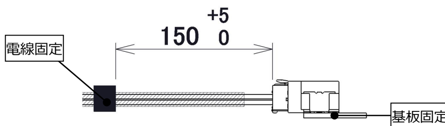
図 9. 固定方法
