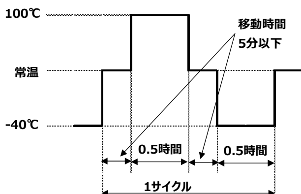
図 6.サーマルショック
