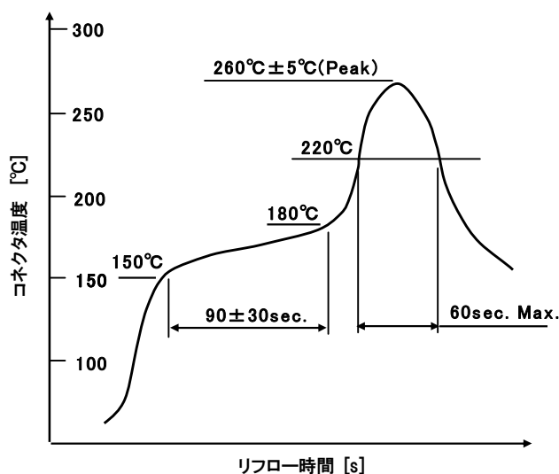
図 1.リフロー温度プロファイル
