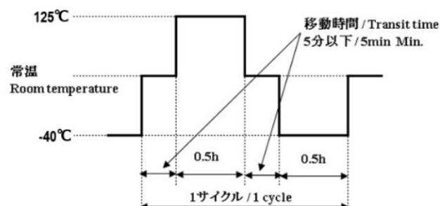
図 3 サーマルショック温度パターン
