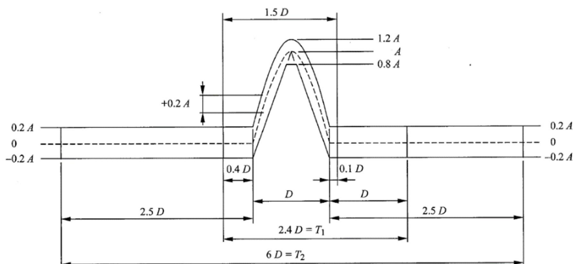
図 7 半正弦波
