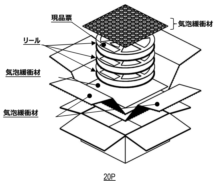
図 1.エンボスリール
