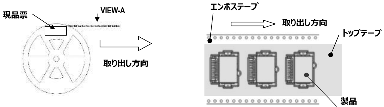
図 1.エンボスリール
