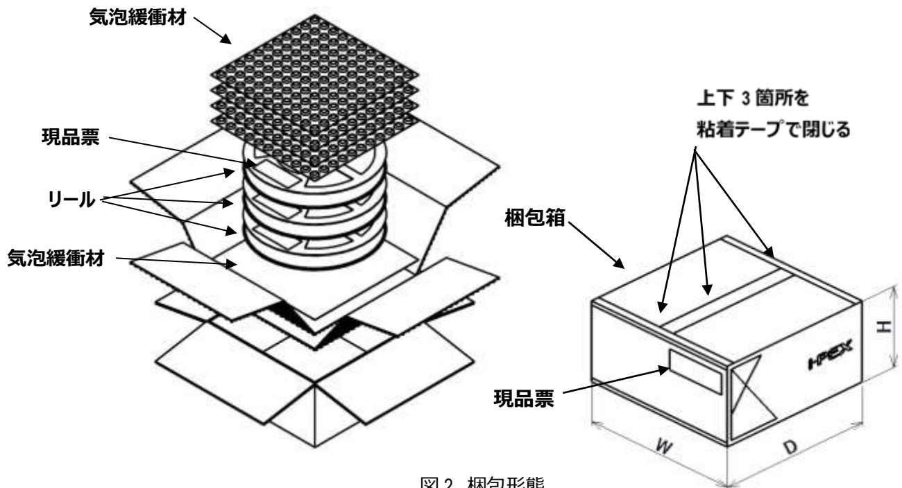
図 2. 梱包形態
