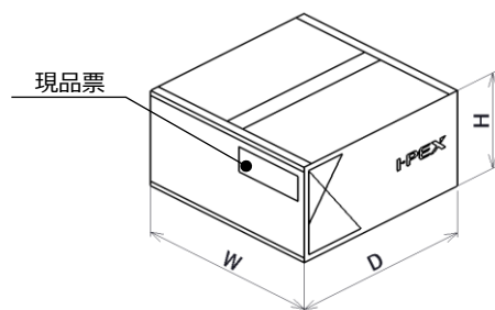
図 4. 外箱
