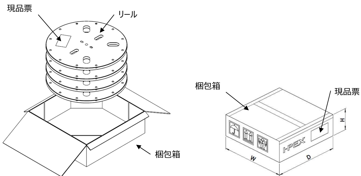
図 2. 梱包形態
