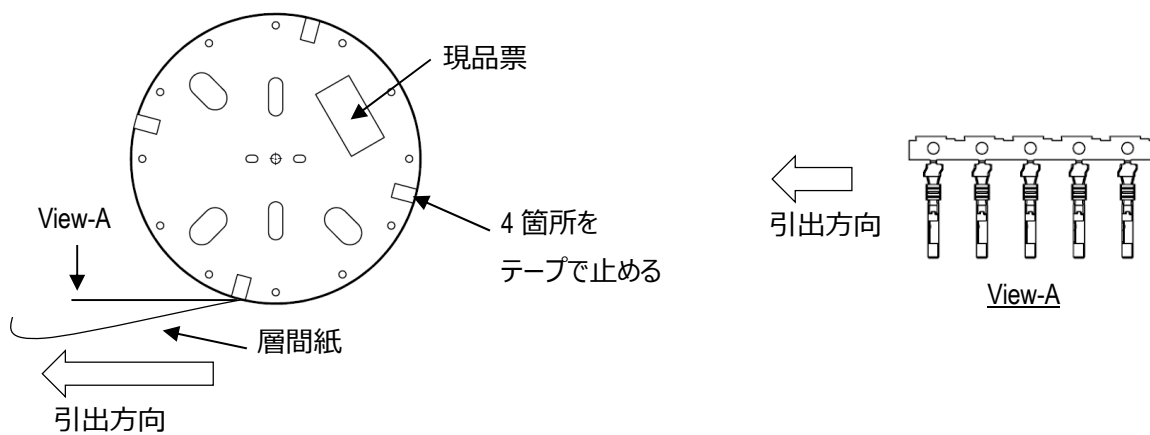
図 1. リール
