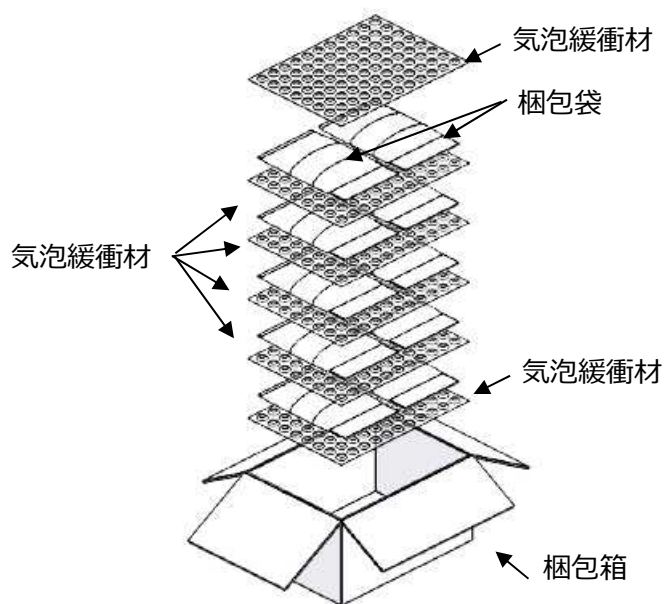
図 3. 梱包形態
