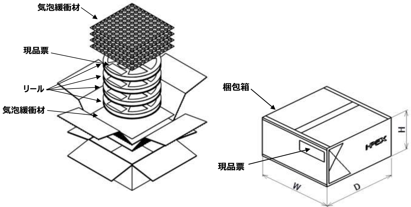
図 2. 梱包形態
