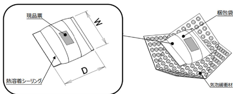
図 2 梱包袋
