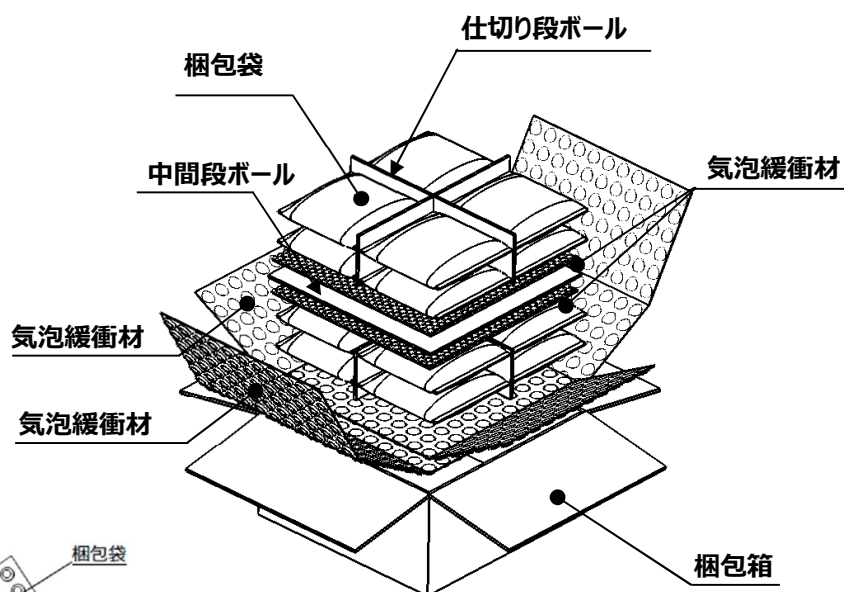
図 3 梱包形態
