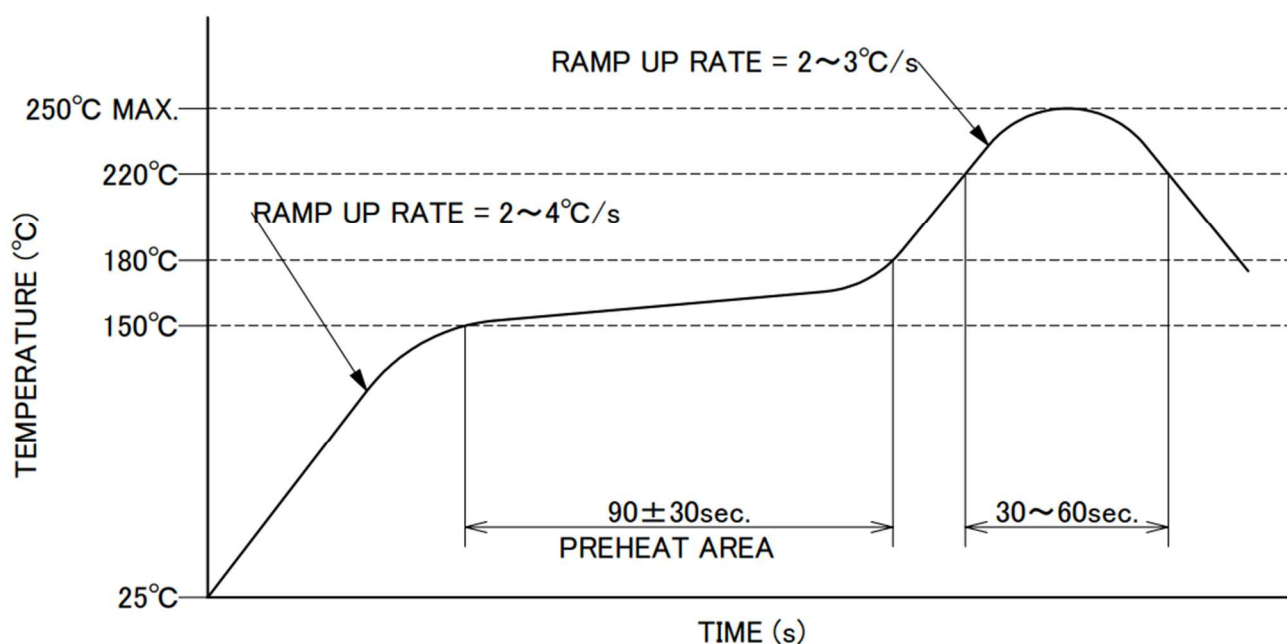
推奨リフロー温度プロファイル
