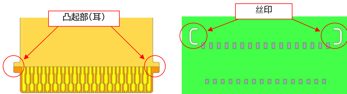
图 5. FPC 插入确认用(参考)
