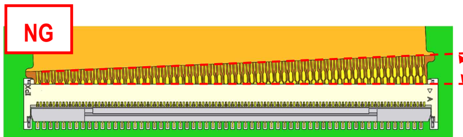
NG-② : Oblique insertion
