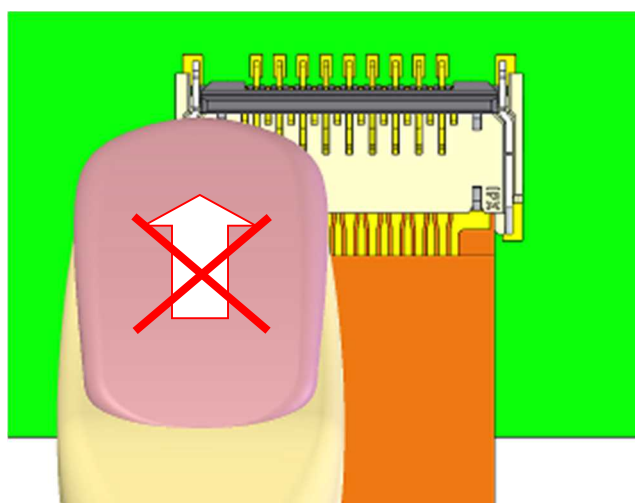
図 11. アクチュエータのクローズ方法 (NG) / Fig.11 To close actuator (NG)
