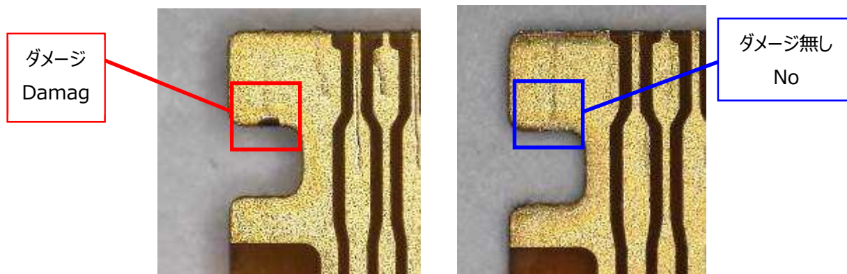
図. 21(a) アクチュエータクローズ状態で抜去した場合(b) 正常抜去した場合
