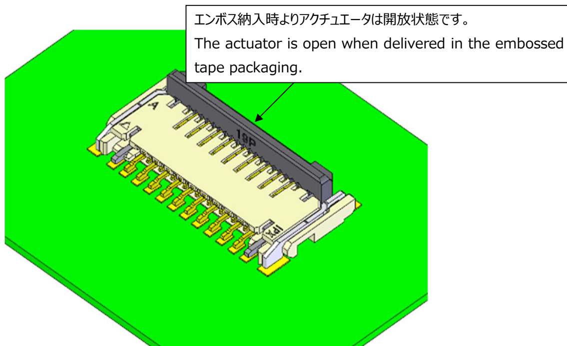
図 2. コネクタ実装状態 / Fig.2 Connector mounting state
