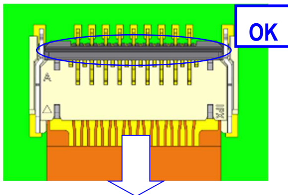
図 18. FPC の抜去方法 (OK) / Fig.18 To withdraw FPC (OK)
