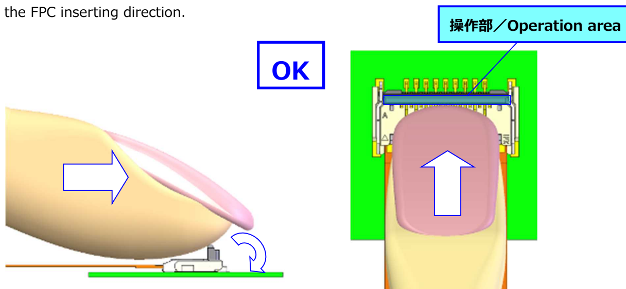
図 9. アクチュエータのクローズ方法 (OK) / Fig.9 To close actuator (OK)
