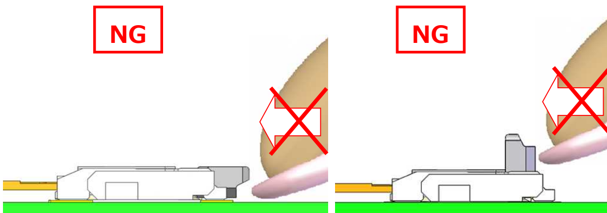
図 16. アクチュエータの解除方法 (NG) / Fig.16 To release actuator (NG)
