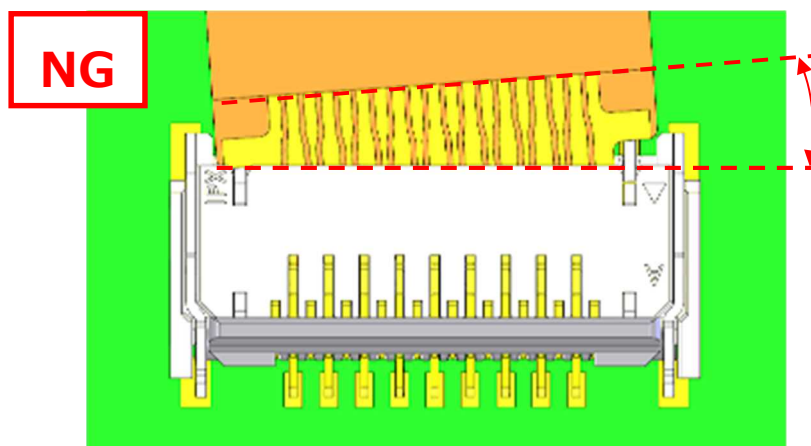
図 4. FPC 挿入方法 (NG) / Fig.4 FPC insertion (NG)
