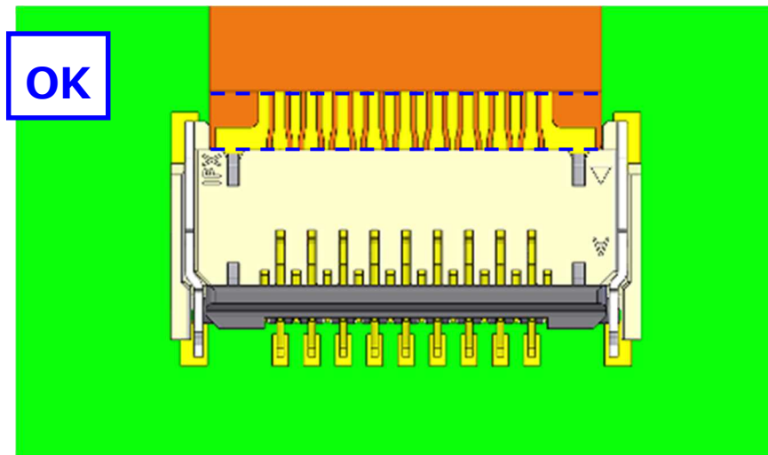
図 3. FPC 挿入方法 (OK) / Fig.3 FPC insertion (OK)
