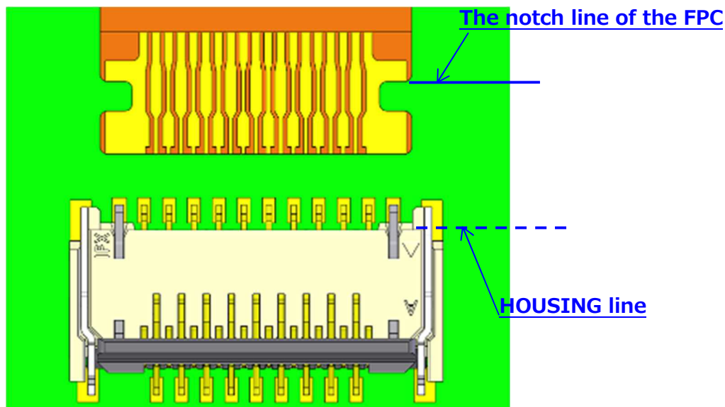
図 5. FPC 挿入方法 / Fig.5 FPC insertion
