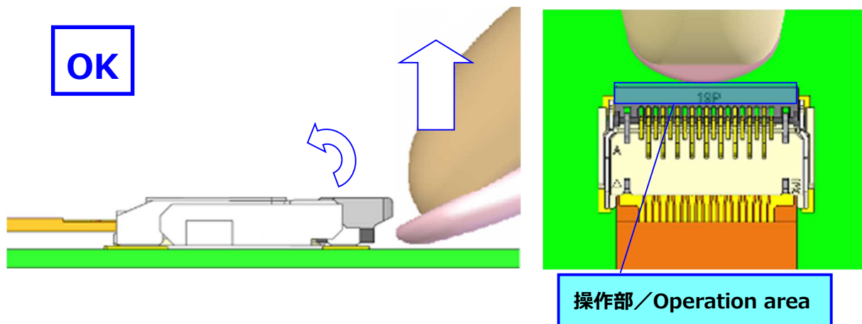
図 14. アクチュエータの解除方法 (OK) / Fig.14 To release actuator (OK)
