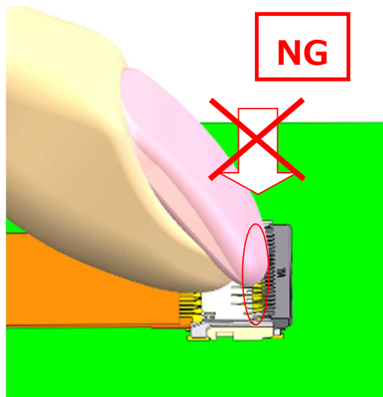
図 12. アクチュエータのクローズ方法 (NG) / Fig.12 To close actuator (NG)
