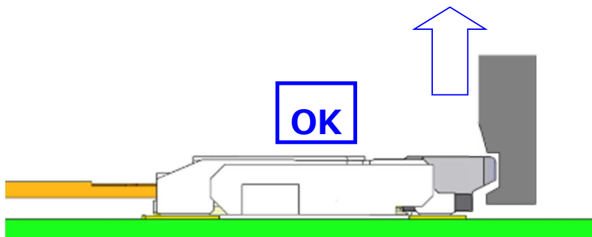
図 15. アクチュエータの解除方法 (OK) / Fig.15 To release actuator (OK)
