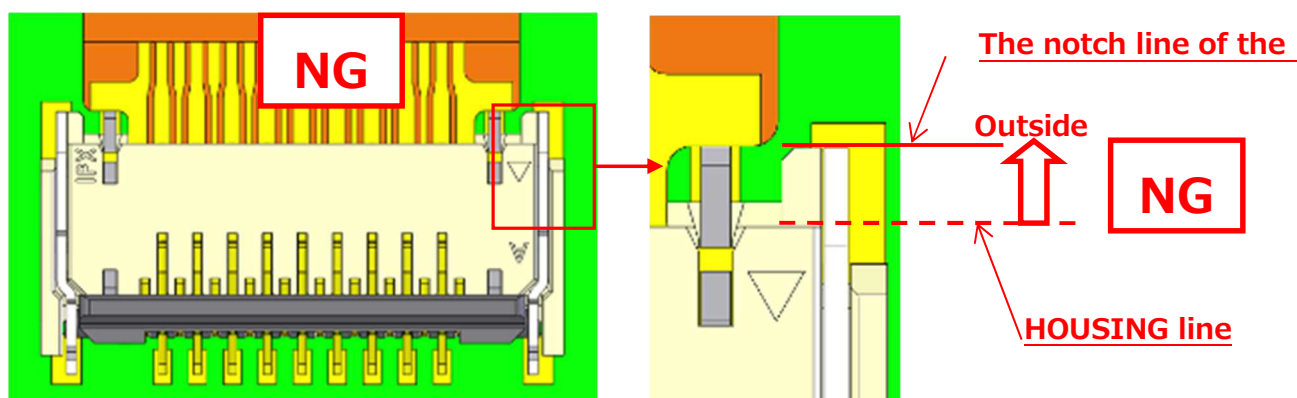
図 7. FPC 挿入方法 (NG) / Fig.7 FPC insertion (NG)
