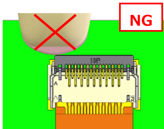
図 17. アクチュエータの解除方法 (NG) / Fig.17 To release actuator (NG)
