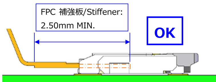
図 22. FPC の屈曲 (OK) / Fig.22 Flexion of FPC (OK)
