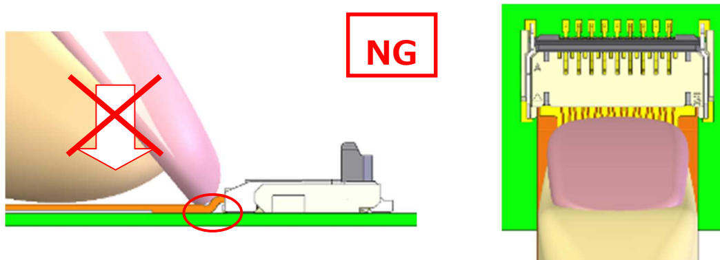
図 8. FPC 挿入方法 (NG) / Fig.8 FPC insertion (NG)
