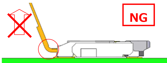
図 23. FPC の屈曲 (NG) / Fig.23 Flexion of FPC (NG)
