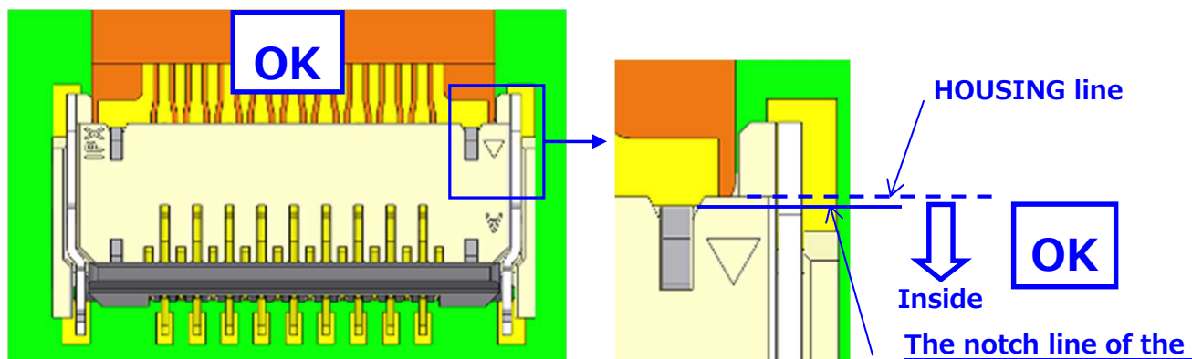
図 6. FPC 挿入方法 (OK) / Fig.6 FPC insertion (OK)
