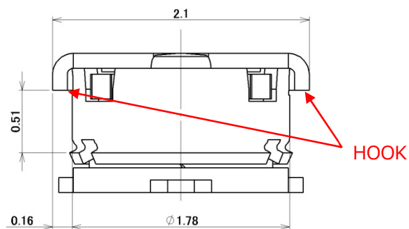
Fig. 2 抜去 JIG 引っ掛け形状配置図
