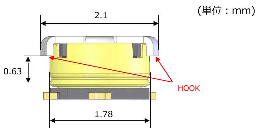
(Fig. 2) 抜去 JIG 引っ掛け形状配置図
