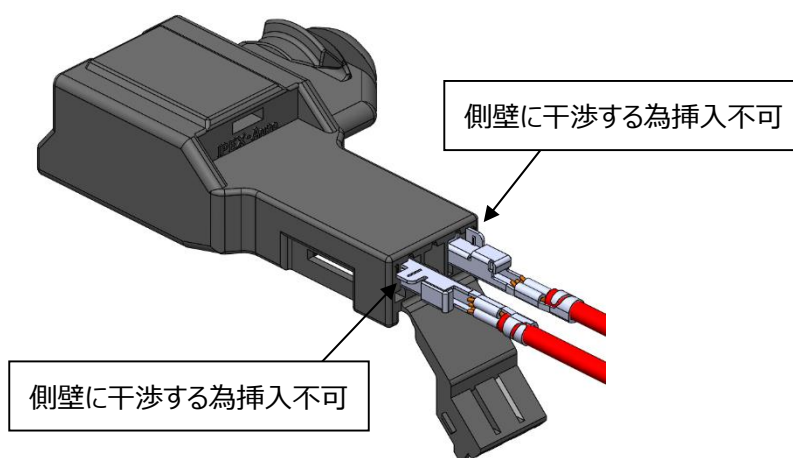
図 25.端子逆挿入
