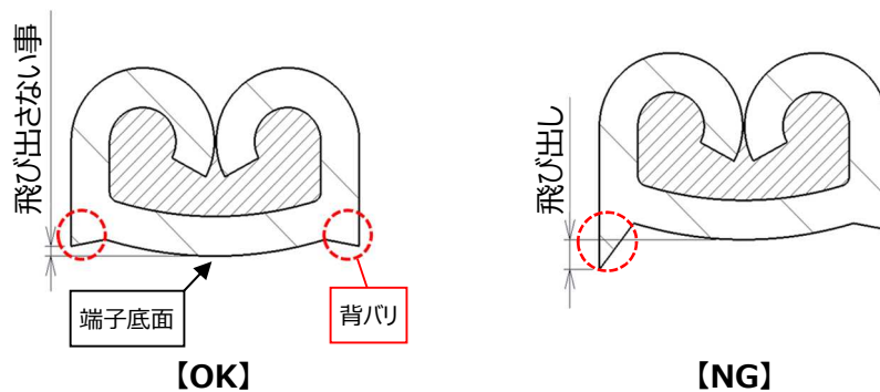
図 9. 背バリ
