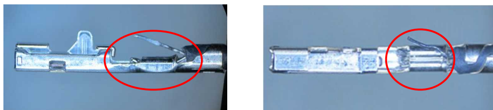
図 20.芯線はみ出し状態
