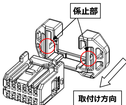
図 48. リヤカバー取付け方向
