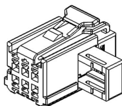
図 35.リテーナ逆挿入状態
