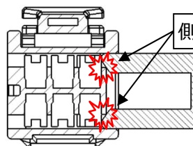
図 35.リテーナ逆挿入状態
