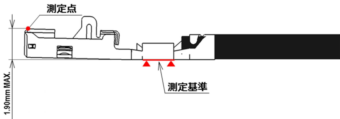
図 15.ベンドアップ
