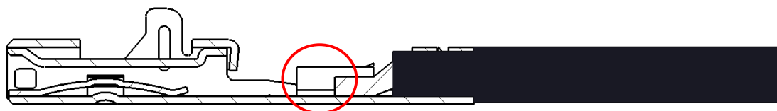
図 18.芯線挿入不足状態
