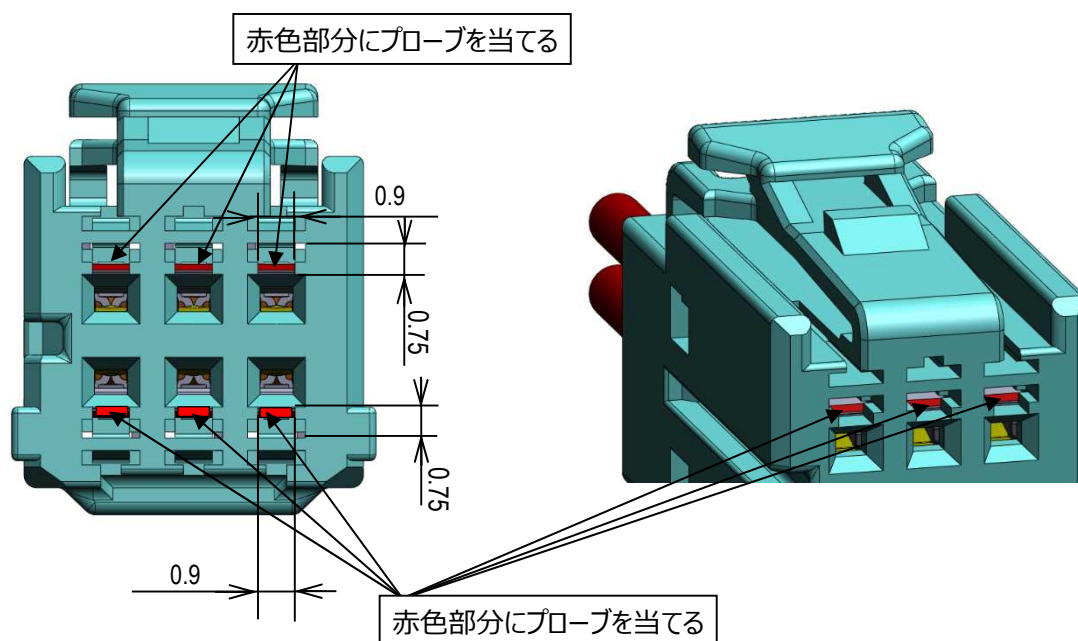
図 55. メスコネクタ導通検査接点
