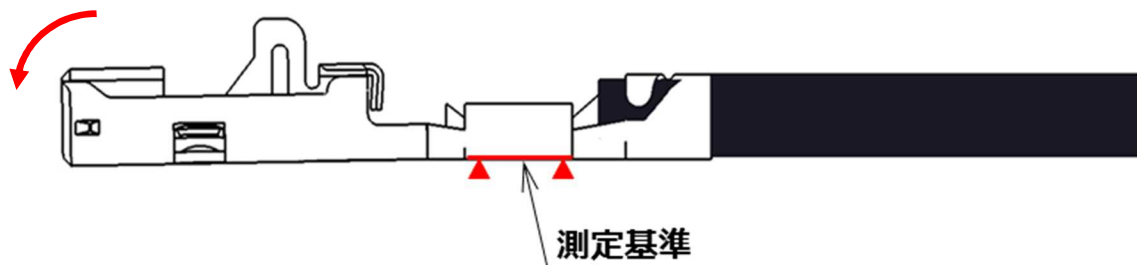
図 16.ベンドダウン
