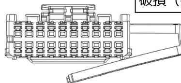
図 34.リテーナ非正規挿入
