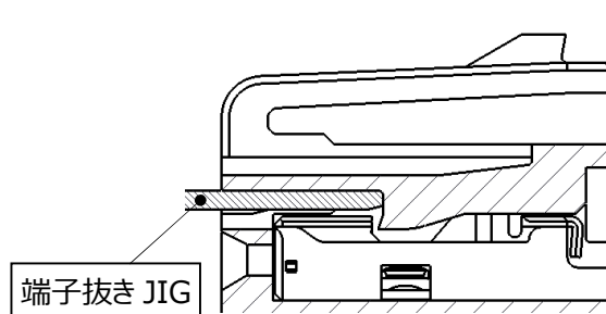
図 39.抜き JIG が樹脂ランスに突き当たる位置
