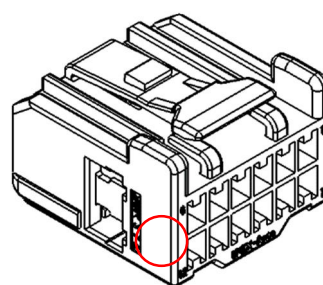
図 45. リヤカバー非対応メスハウジング
