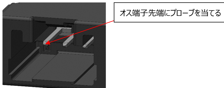
図 52. オス端子導通検査接点
