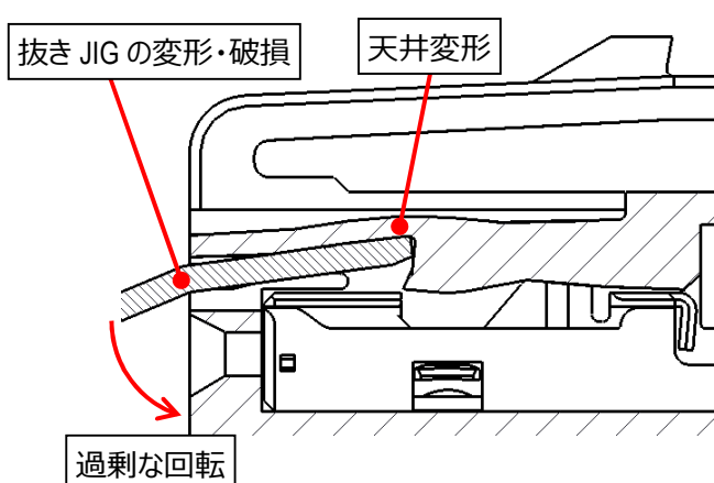
図 42. 天井変形、抜き JIG の変形・破損
