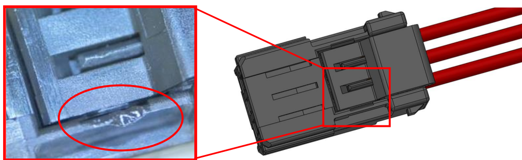
図 31. 二次係止部保持部傷例
