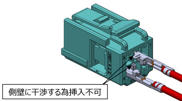
図 27.メスハウジング端子誤挿入
