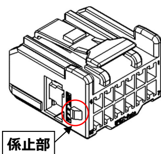
図 44. リヤカバー対応メスハウジング
