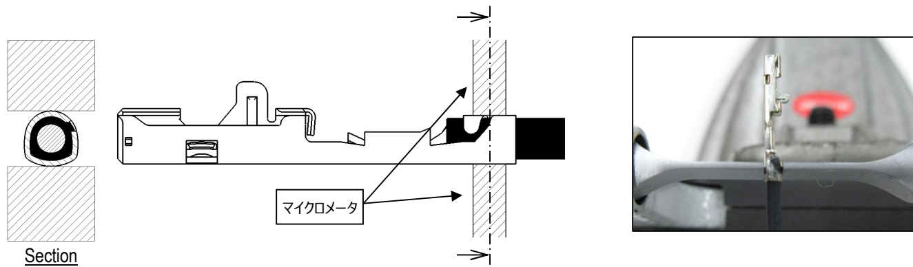
図 6.インシュレーションバレルクリンプハイト測定方法
