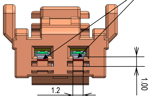
図 53.メス端子導通検査接点
