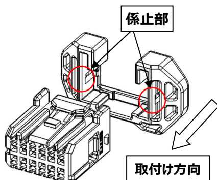
図 46. リヤカバー取付け方向
