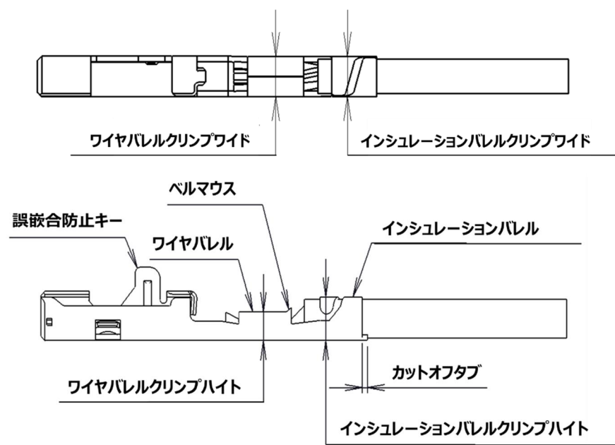
図 3.端子各部名称
