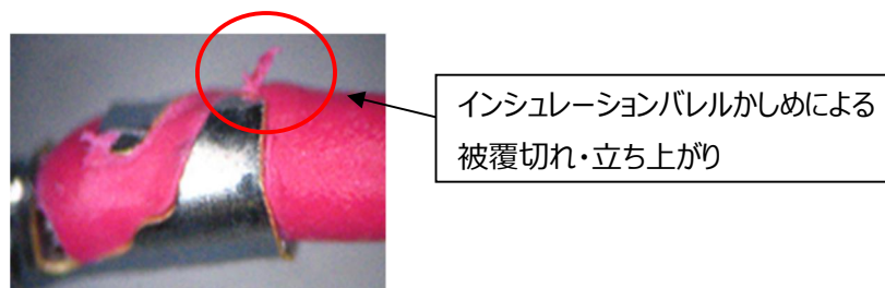
図 24.被覆切れ状態
