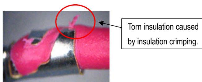
Fig 24. Torn insulation
