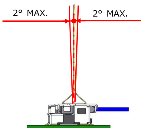
Fig.35 PULL TAPE でのこじり許容角度
