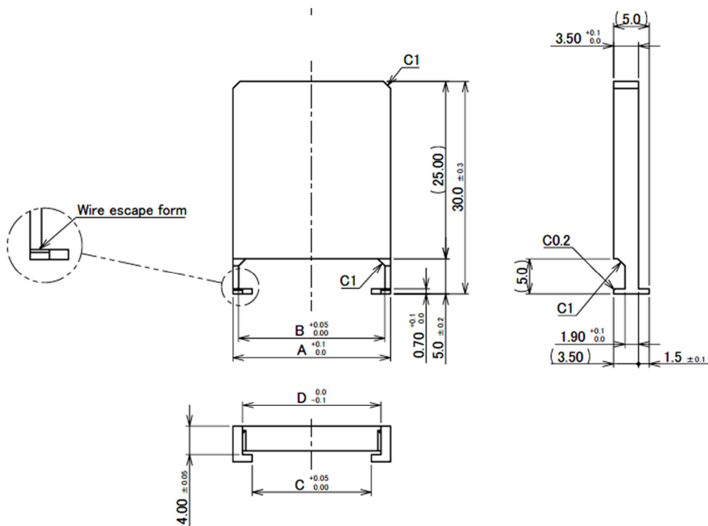
Fig.25 参考 抜去 JIG
