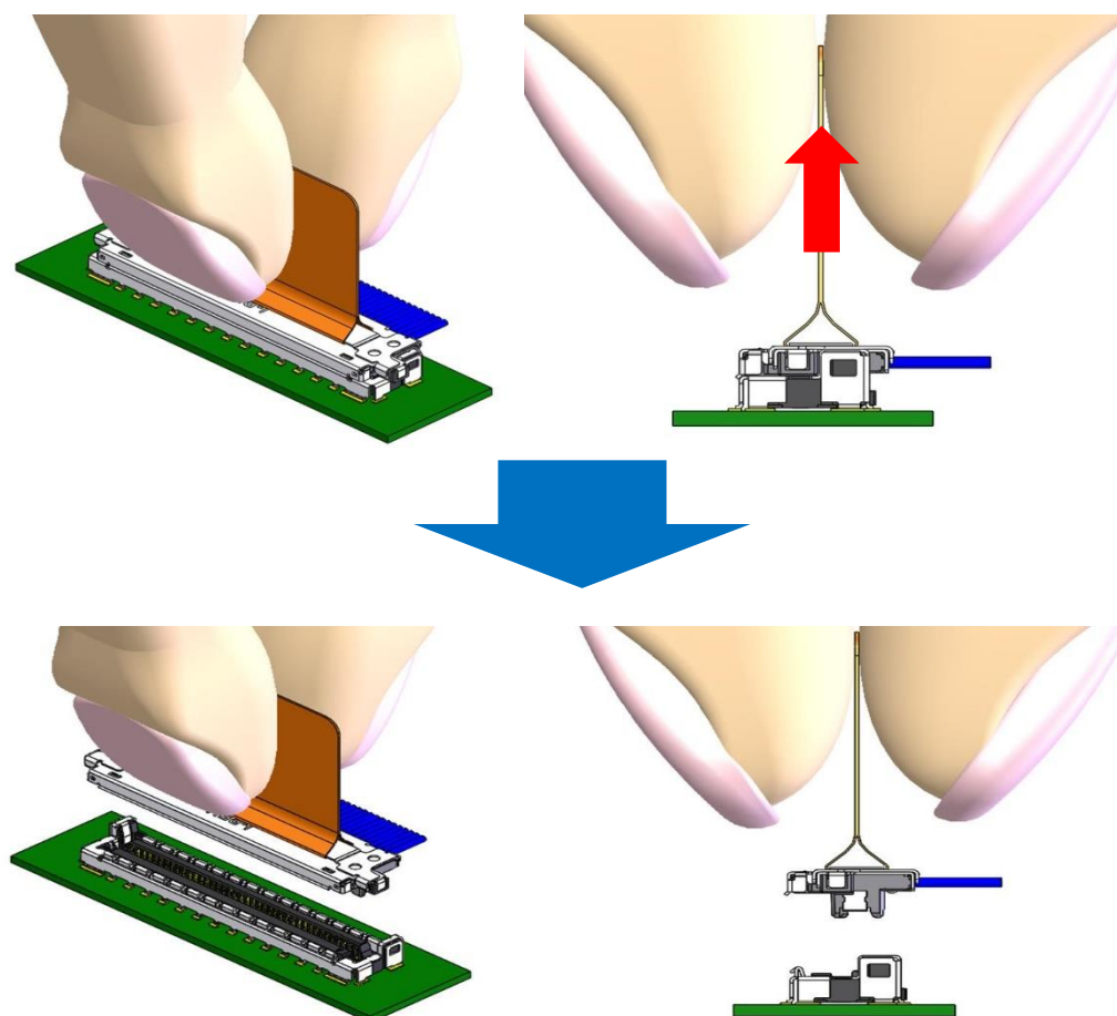
图.32 利用 Pull Tape 拔出的方法
