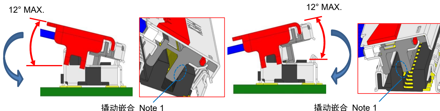
图.8 允许插入角度
