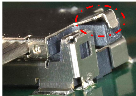
照片.2 Shell-A 变形
