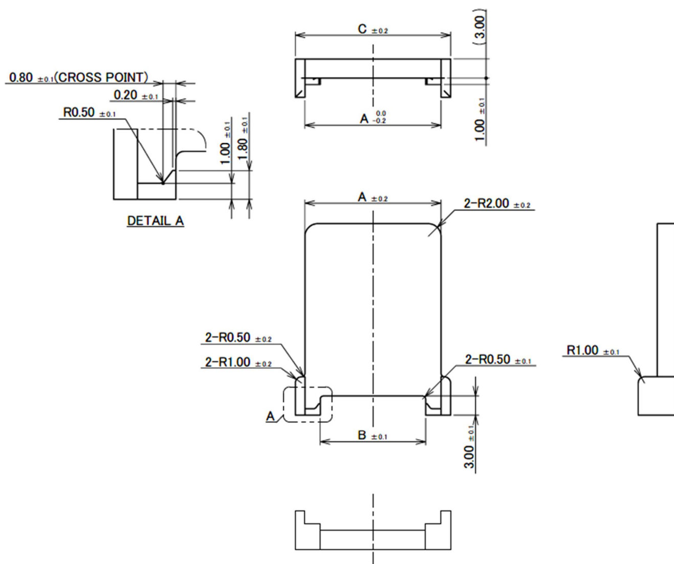
图.24 参考 解锁 Jig
