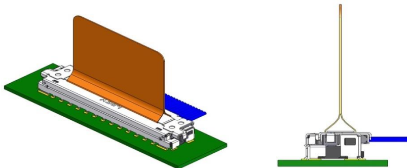
图.31 有 Pull Tape 的嵌合状态
