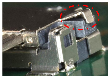
照片.1 Shell-A 变形
