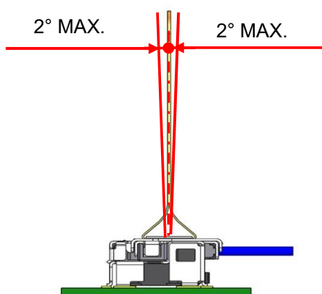
图.35 利用 Pull Tape 时的允许撬动角度
