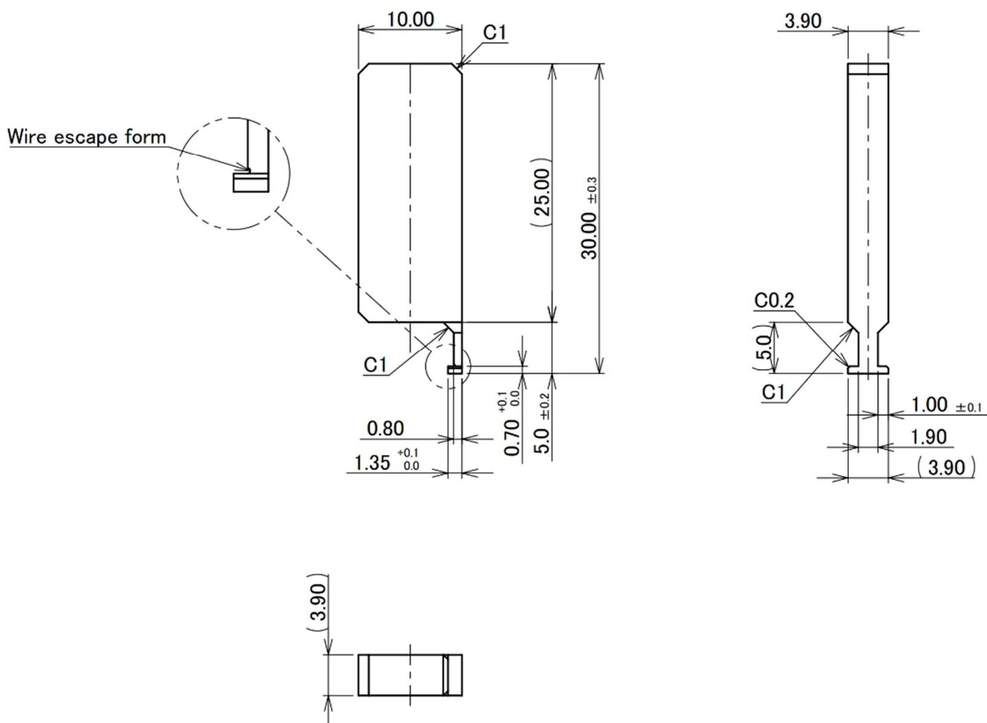
图.26 参考 单侧拉拔 Jig
