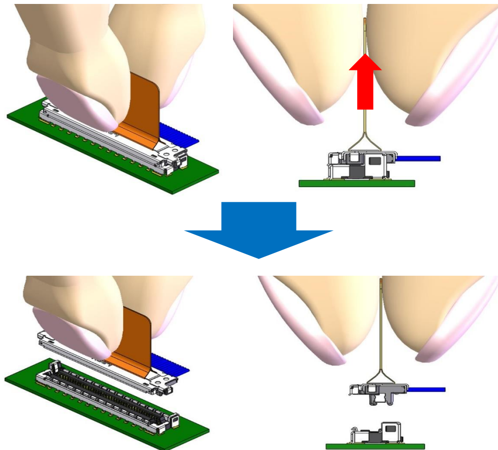
Fig.26 利用 PULL TAPE 拔出的方法
