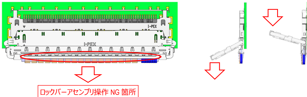
図. 22 抜去 NG 行為 1
