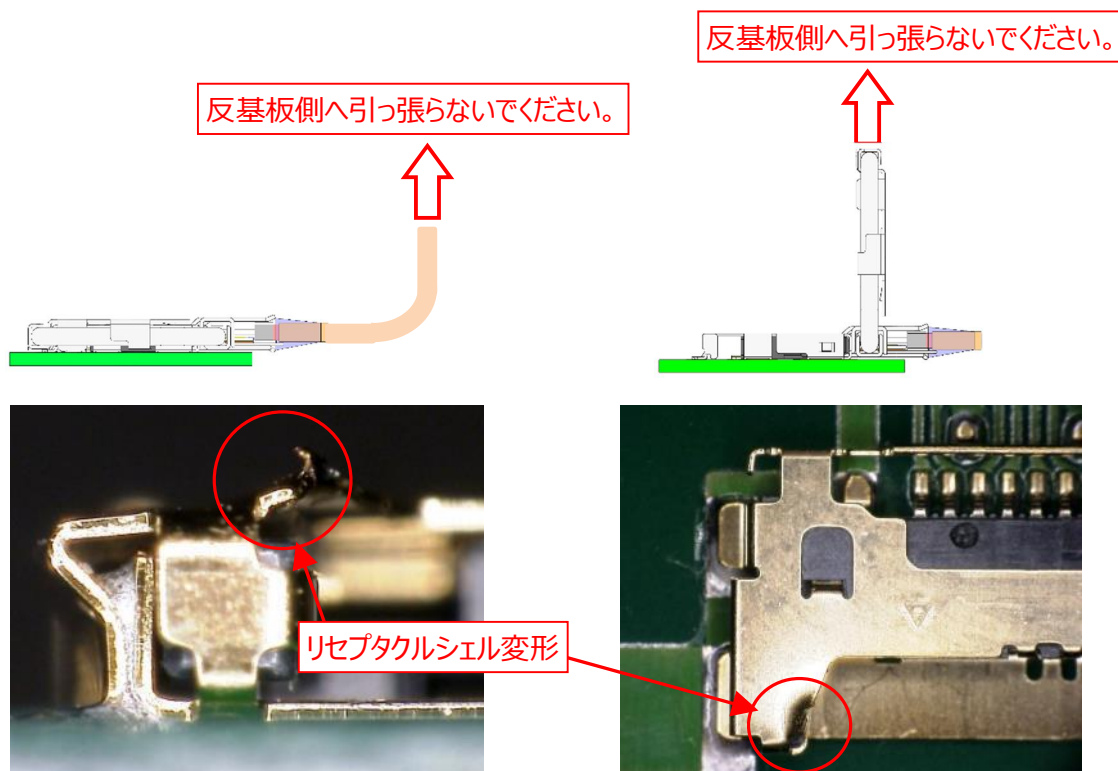
図. 24 Harness とロックバーアセンブリの操作 NG 行為
