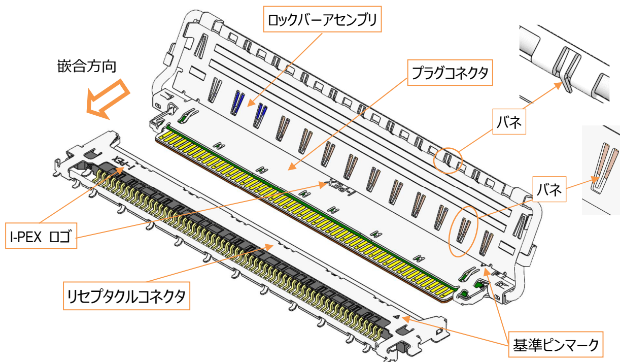
図. 3 コネクタ各部名称
