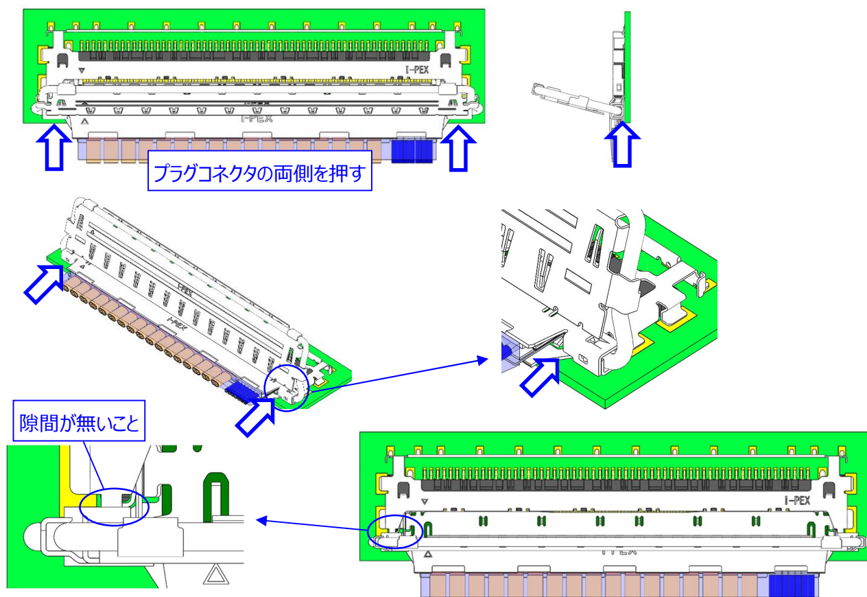
図. 5 プラグコネクタ挿入方法
