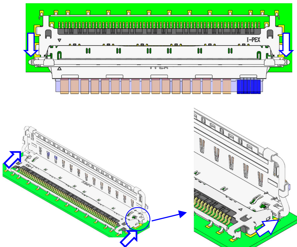
図. 20 抜去操作箇所
