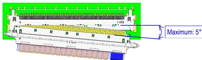
図. 21 水平方向 最大抜去角度
