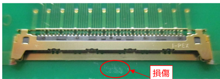
図. 14 挿入 NG 行為 2
