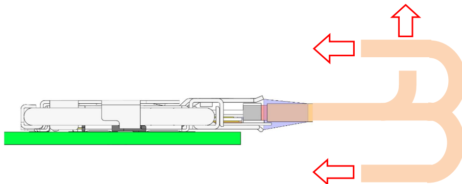
図. 25 ケーブルの引き回し NG 方向
