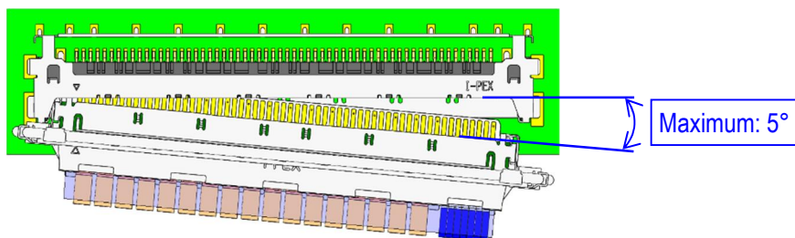
図. 10 水平方向 最大挿入角度
