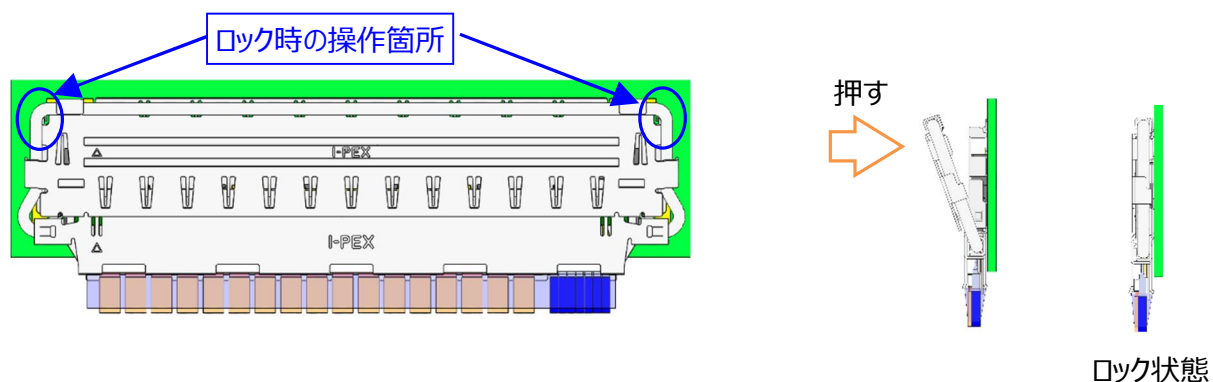
図. 15 嵌合ロック方法
