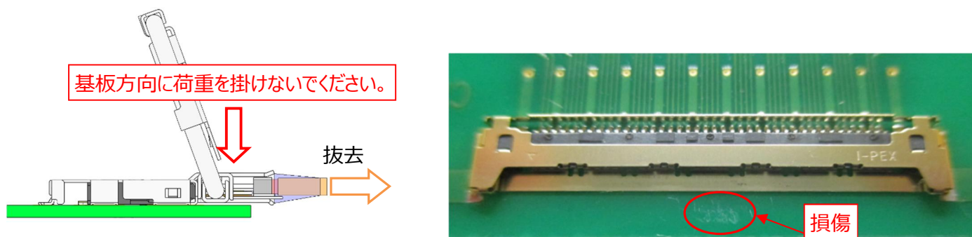
図. 23 抜去 NG 行為 2
