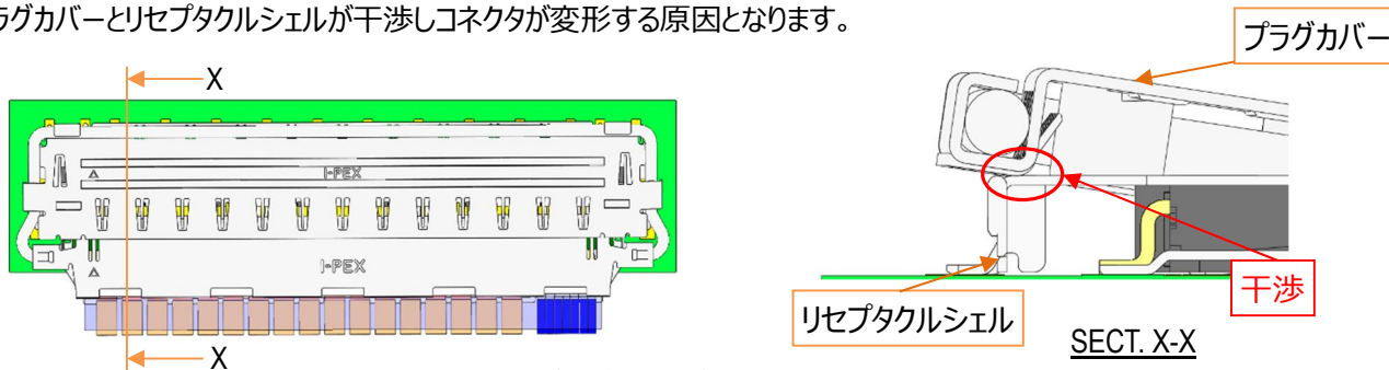
図. 7 プラグとリセプタクルコネクタの干渉
