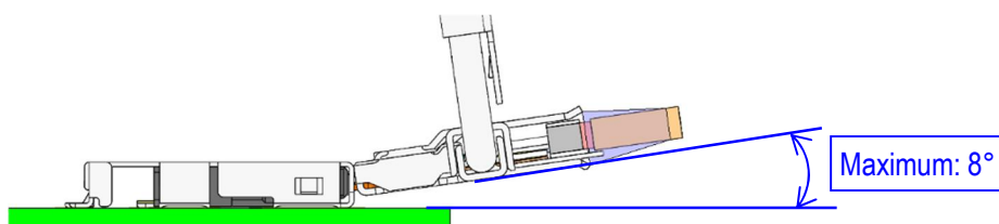
図. 82 垂直方向 最大挿入角度
