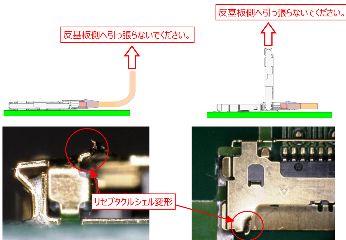
図. 25 Harness とロックバーアセンブリの操作 NG 行為
