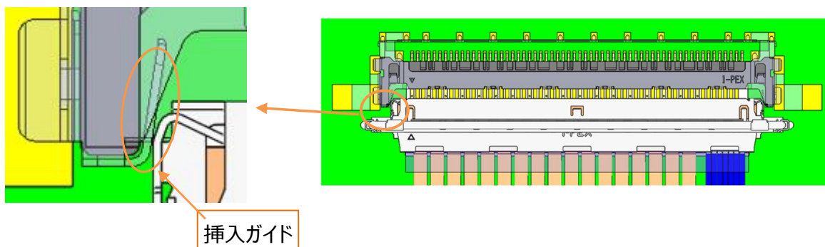
図. 8 挿入ガイド
