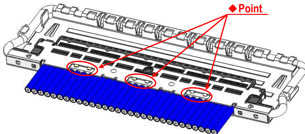
図 12. SHELL-B 及び GND BAR 半田付け箇所
