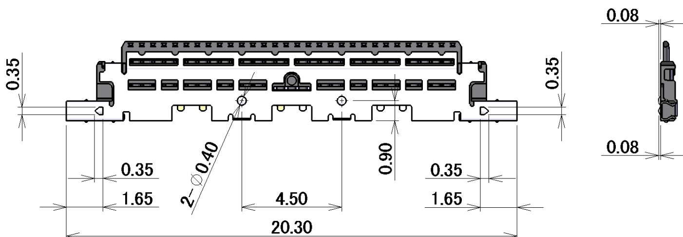
図 4. PLUG HSG ASS'Y SHELL 底面側
