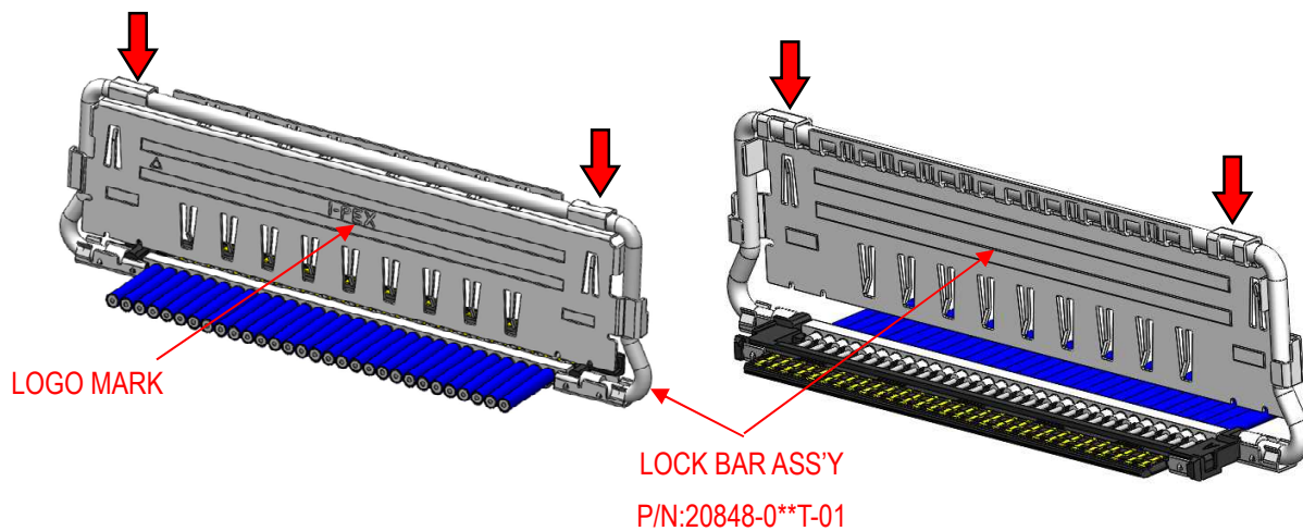
図 6. LOCK BAR ASS'Y 組み付け方法
