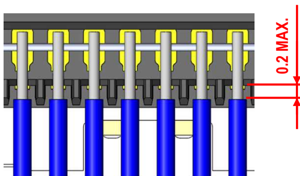
図 3. ディスクリートケーブルセット位置
