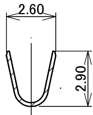
SECTION A-A
