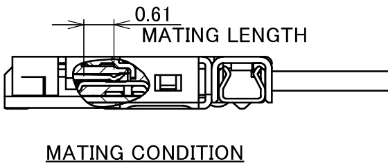
SECT.X-X (S=10:1)
