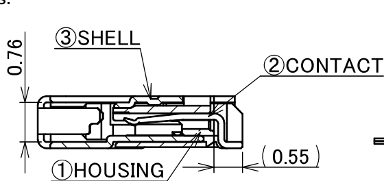
SECT.X-X (S=10:1)
