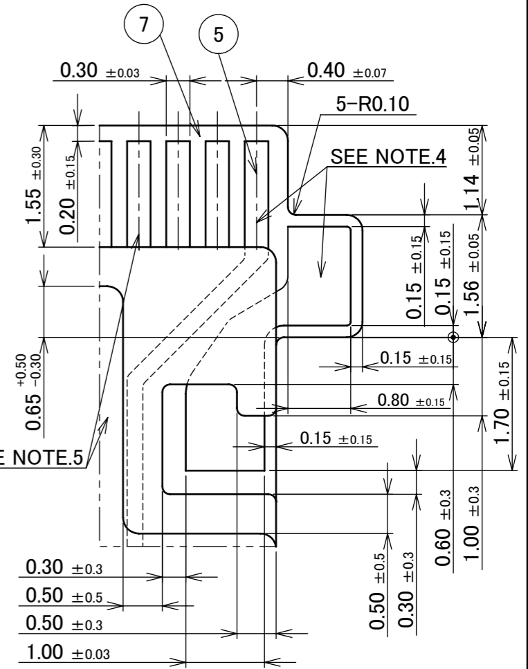
DETAIL DD (S=15/1)
