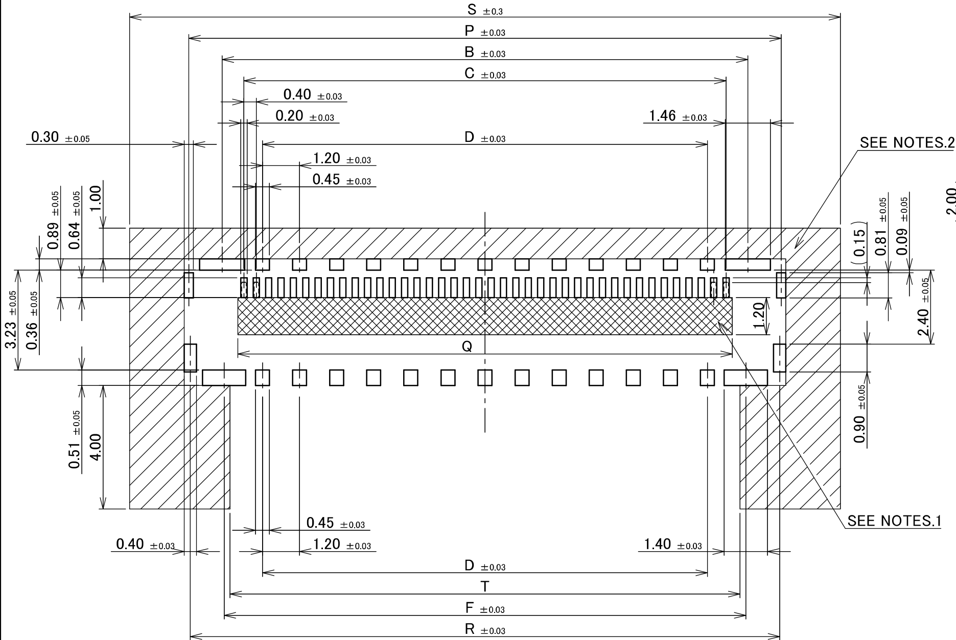
RECOMMENDED PCB LAYOUT 【TYPE A】 (S = 8 : 1)
