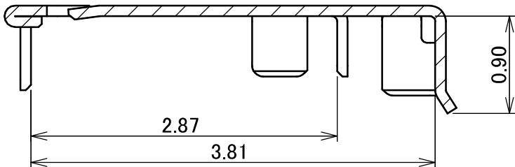
SECT.AA-AA (S=20/1)
