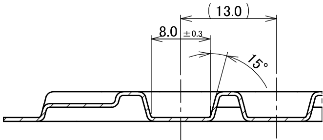
SECT.Y-Y (S=2/1)
