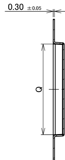
SECT EE-EE (S=2 : 1)
