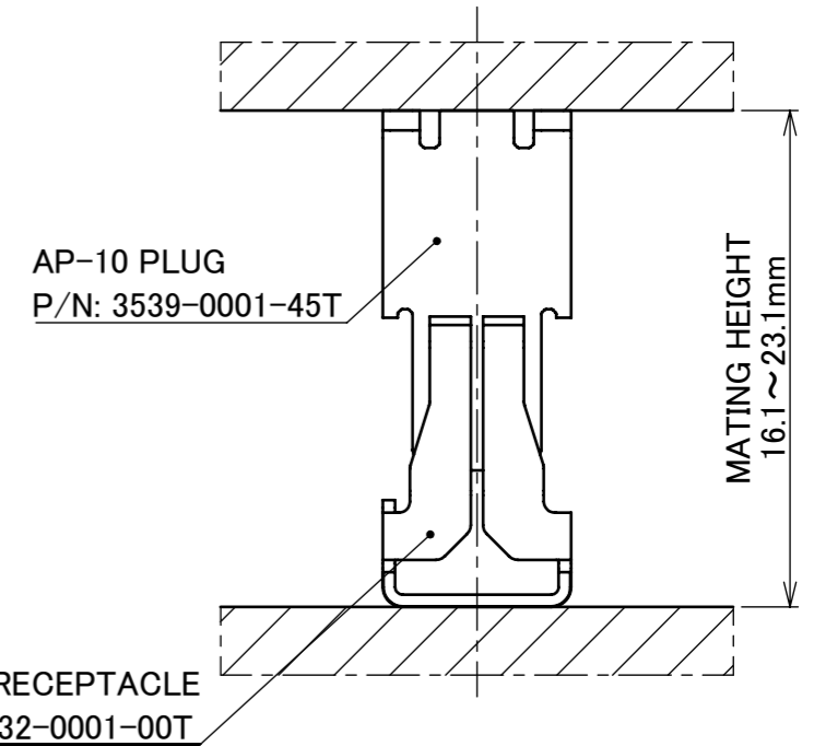
MATING CONDITION 【AP-10 PLUG H=14.5 mm】
